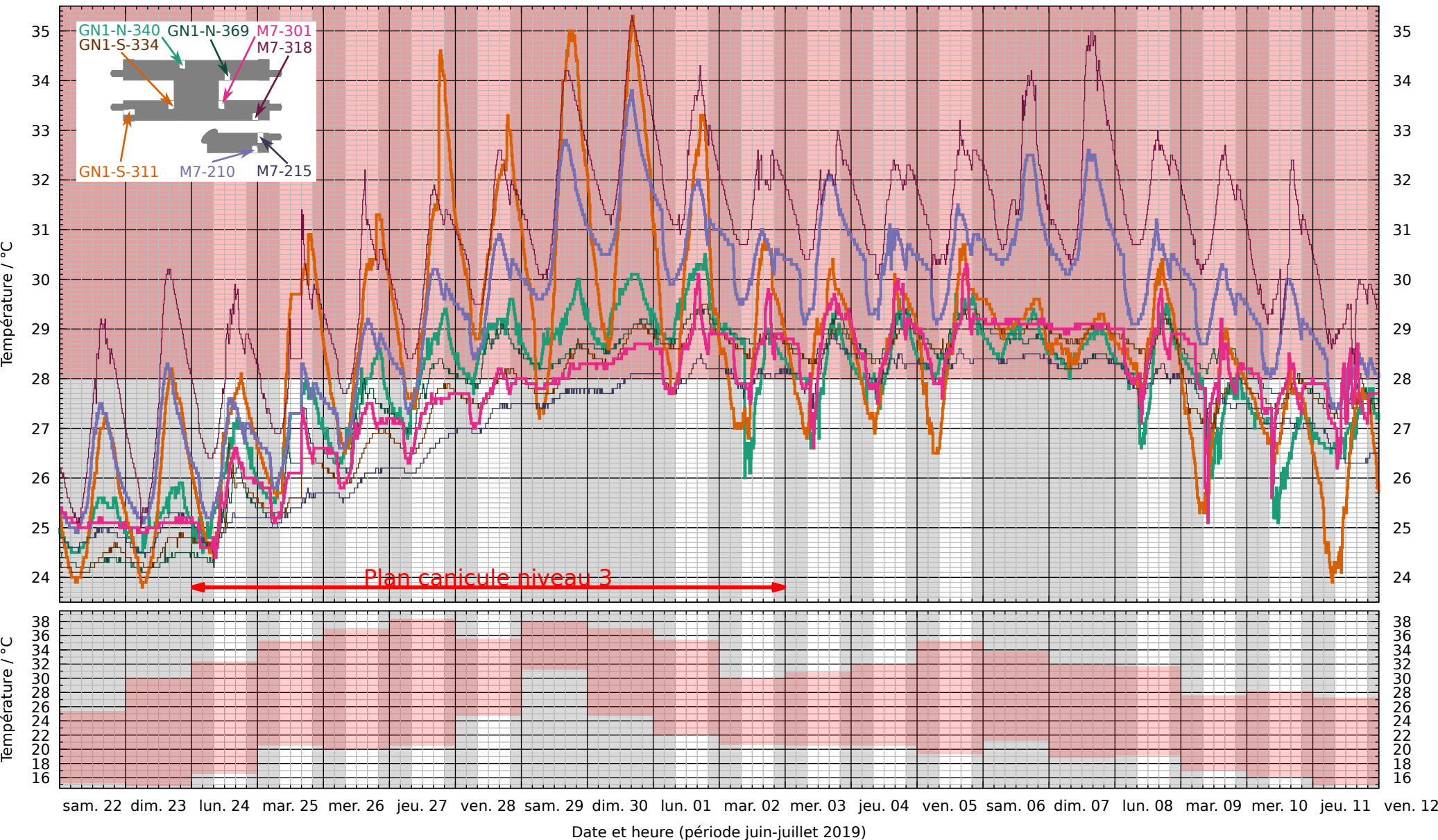
Relevés de température dans les bureaux du LIP et dans la station météo du site Descartes
