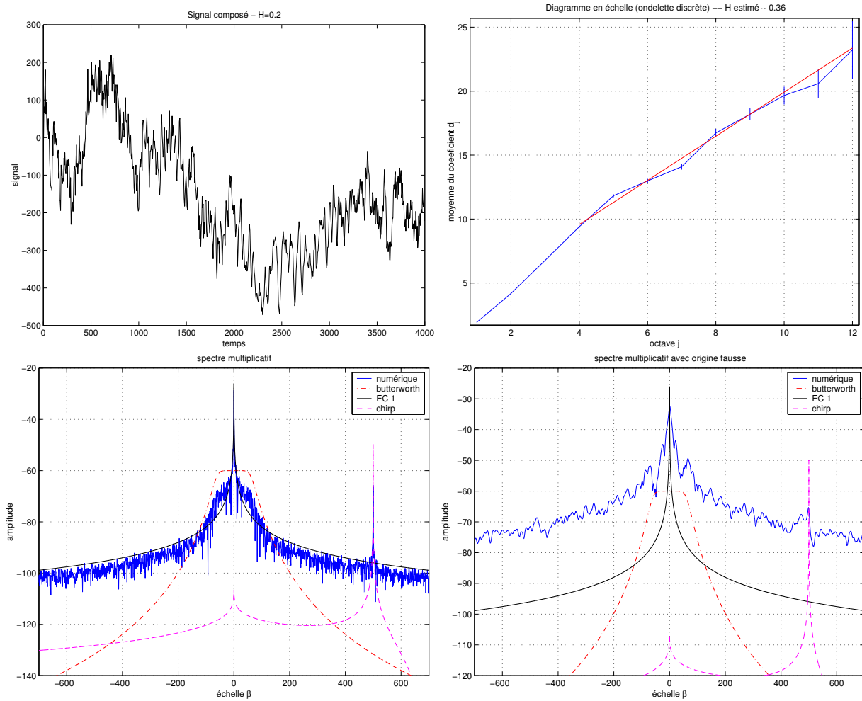
Fig. II.26: Signal formé par l'addition de la sortie d'un EC d'ordre 1, du signal de spectre type Butterworth de la figure II.25, d'un chirp de Mellin H = 0.2 et \beta_0 = 500 et de bruit blanc Gaussien à -80 dB. À l'exception du bruit le processus est exactement H -ss (théoriquement et propriété obtenue aussi numériquement). Cependant la struture auto-similaire complexe perturbe l'estimation de l'exposant (en haut à droite) qui par décomposition en ondelettes discrètes se voit attribué l'estimation H \simeq 0.36 \pm 0.04 . En bas on montre comment le spectre de Mellin d'une réalisation, sans moyenne (en bas à gauche) rend compte des propriétés du signal synthétisé, mais aussi que la connaissance de l'origine est cruciale pour cette analyse (en bas à droite, TMD avec une erreur de 1% sur la détermination de l'origine).
