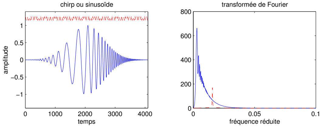
Fig. III.2: Alors que pour une sinusoïde (en - -) la transformée de Fourier est une description suffisante, pour un chirp (en —) elle ne délivre pas toute l'évolution non stationnaire du signal.
