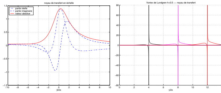
Fig. V.8: Graphe des noyaux de transfert en échelle. À gauche n'est représentée que la fraction \frac{n(2\pi\gamma+2\pi\beta-2i)}{(2-i2\pi(\beta-\gamma))^2} , tandis qu'à droite on a pris Z_0(\beta) = (1 + ih\pi\beta)\Gamma(i\pi\beta)/2 . Sur ce deuxième graphe on montre les cas pour \beta = n2\pi avec n allant de 1 à 3. On constate que le transfert est principalement local (autour de \beta = 0 sur la graphe de gauche et de \gamma = \beta à droite) en échelle.
