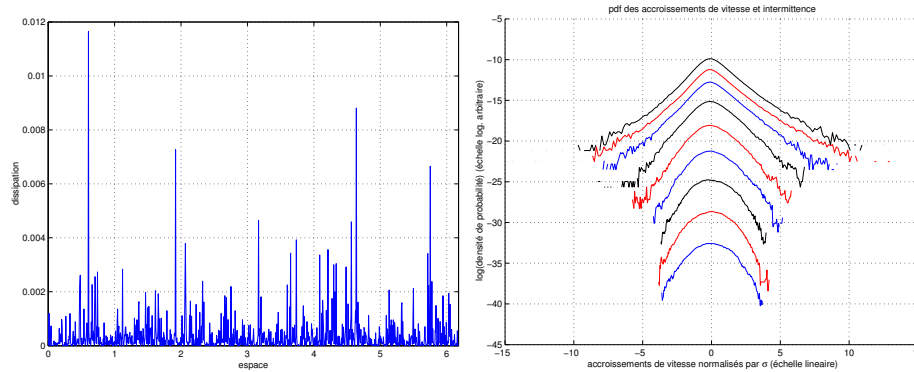
Fig. V.2: À gauche, estimation de la dissipation locale associée au signal de vitesse de la figure V.1. L'intermittence est ici associée à l'existence de bouffées d'activité irrégulières. À droite, l'estimation des densités de probabilité des accroissements de vitesse à différentes échelles est responsable d'une intermittence qualifiée de statistique. Le graphique est en semi-log, les courbes sont arbitrairement décalées pour la lisibilité et à grande échelle ressemblent à une distribution gaussienne pour développer des ailes exponentielles de plus en plus marquées quand l'échelle diminue (courbes du haut).
