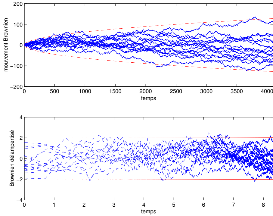
Fig. 11.3: Illustration de la transformée de Lamperti : en haut sont représentées différentes réalisations de mouvement Brownien, où l'évolution de deux fois la variance est indiquée en trait - -, tandis qu'en-dessous on montre les processus stationnaires délampertisés qui restent confinés principalement entre les deux traits mis à 2 fois la variance du processus.
