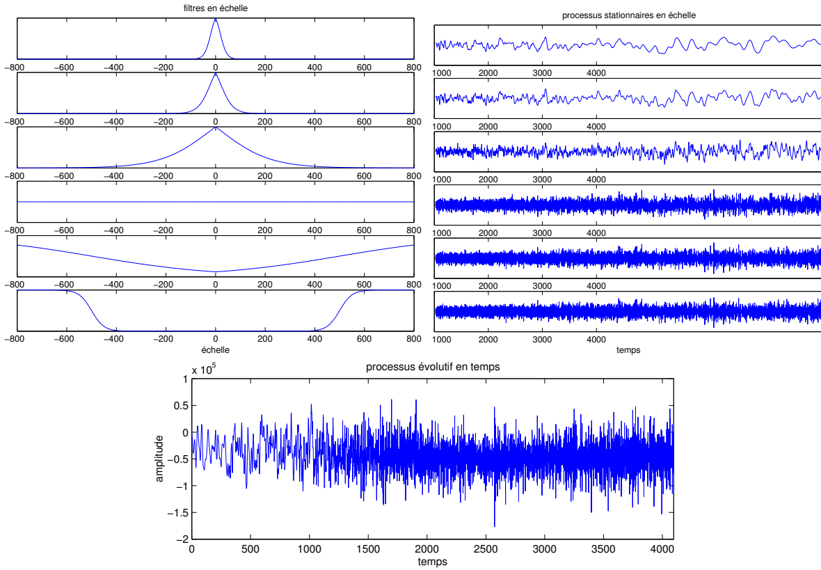
Fig. III.5: Synthèse d'un processus qui n'est pas auto-similaire mais a des propriétés qui évoluent continuellement en échelle au cours du temps (voir le texte). La batterie de filtres utilisés et des exemples de leur comportement auto-similaire sont donnés au-dessus. En faisant glisser le comportement du filtre multiplicatif instationnaire depuis les filtres passe-bas jusqu'aux passe-haut (en \beta ), nous synthétisons un processus dont le contenu en échelle est de plus en plus riche. Il n'est pas auto-similaire mais sa déviation au H -ss n'est pas une variation de l'exposant en temps, mais de son spectre instantané de Mellin.
