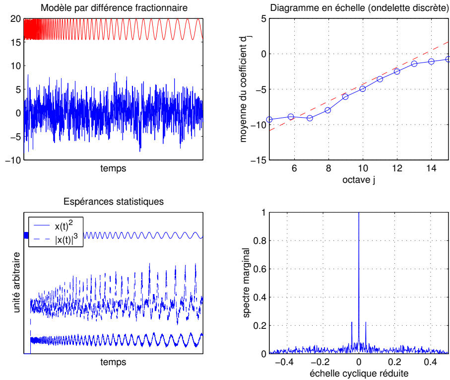
Fig. IV.18: Exemple de réalisation d'un processus à DSI engendré par différence fractionnaire ; H = 0.1 , \lambda = 1.05 . On a superposé au graphe du processus une évolution synchronisée avec le coefficient log-périodique pour référence. En haut à droite on montre le diagramme en échelle qui ici a une pente conduisant à une estimation juste de H égale à 0.1 (processus stationnaire). En bas, nous montrons la DSI à l'aide d'une part de l'évolution de la variance du processus au cours du temps et de son moments d'ordre 3, d'autre part du résultat d'estimation du spectre marginal cyclique sur une réalisation. Les deux pics de part et d'autre du pic central sont bien à la fréquence correspondant à la log-période et sont dans ce cas bien plus repérables. La raison est que le processus ne croissant pas en t^H a moins d'excursions longues loin de zéro et révèle plus facilement les périodicités en échelle.
