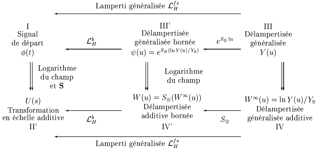
Fig. III.10: Les espaces de représentation de \phi(t) et de sa délampertisée Y(u) ou de sa délampertisée bornée \psi(u) pour les dilatations de taille finie.
