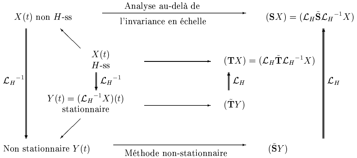
Fig. III.1: Généralisation du cadre de réflexion avec \mathcal{L}_H pour les études des systèmes non invariants.
