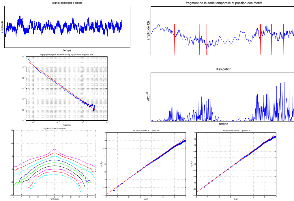
Fig. V.10: Présentation du signal synthétique utilisé pour tester des méthodes d'analyse. Une trace étendue est figurée en haut, tandis qu'un zoom est montré à droite où l'existence de structures autour de certains points est plus visible; en particulier l'équivalent de ce qu'est la dissipation est grande autour de ces points. Ce modèle faux (sans contenu physique) est un bon signal test du fait que son spectre est en k^{-5/3} (spectre au milieu à gauche) et qu'il est intermittent. On montre les distributions des accroissements en bas à gauche et les fonctions S_3(r) et S_4(r) en log-log dont les pentes peuvent être ajustées (en jouant sur les distributions des \alpha ) pour générer l'intermittence voulue.
