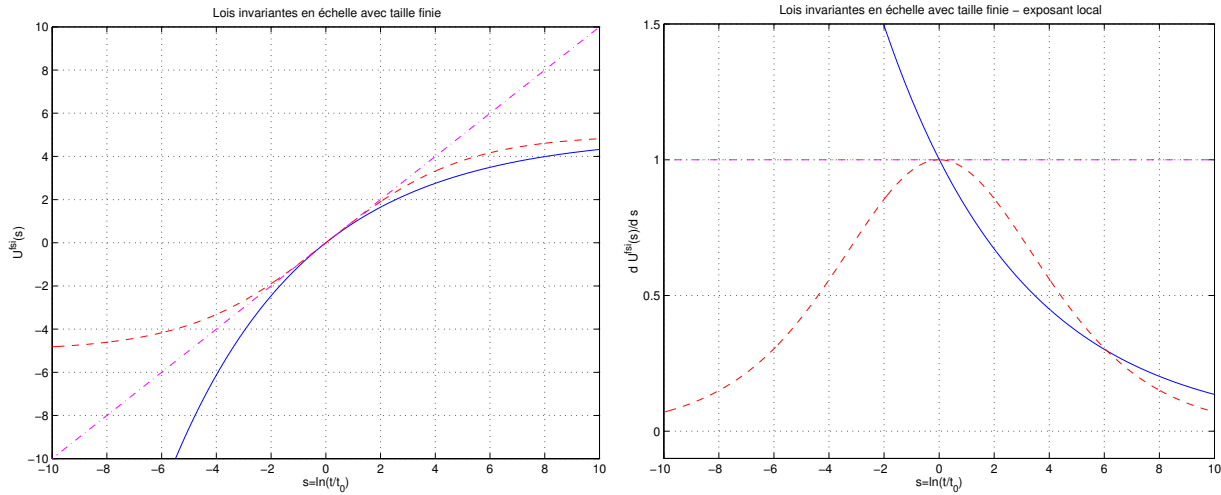
Fig. III.9: Représentation des lois déterministes H -ss avec effets de taille finie ; à gauche on a tracé les lois (en variables log-log), à droite les exposants locaux. Les bornes portent seulement sur le champ ; -- pour deux bornes, - pour une seule P et \cdot - sans limitations.
