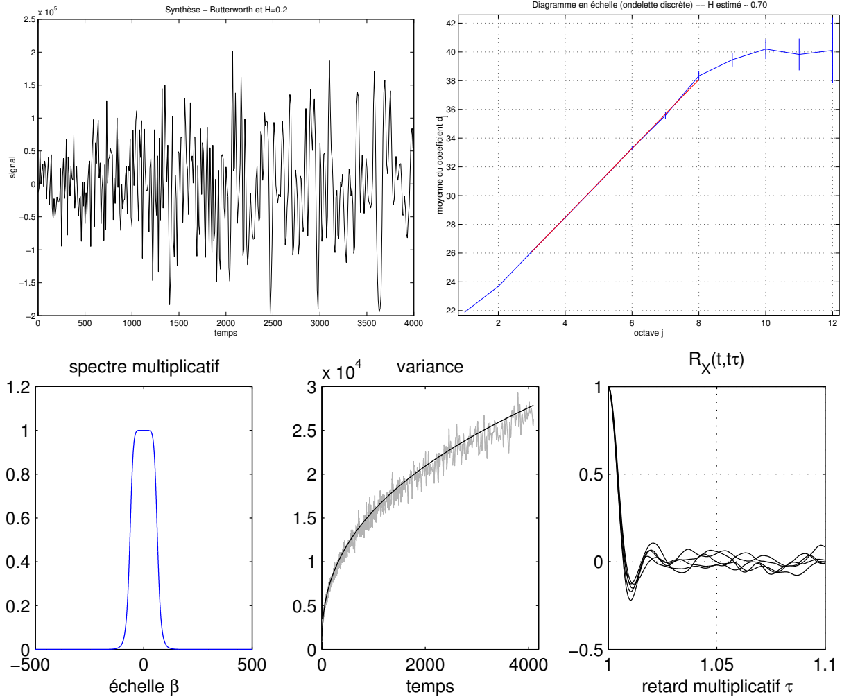
Fig. 11.25: Signal H -ss avec H = 0.2 synthétisé en prescrivant son spectre multiplicatif comme un filtre de Butterworth d'ordre N = 8 et d'échelle de coupure \beta_c = 300 : \mathbf{G}(H + i2\pi\beta) = 1/(1 + |\beta/\beta_c|^N) , représenté en bas à gauche. Une réalisation est montrée en haut à gauche. La variance du modèle estimée sur 1000 réalisations (en bas au centre) obéit à la croissance en t^{2H} et la fonction de corrélation obtenue est représentée en bas à droite comme R_X(t, \tau)/t^{2H} et ne dépend que de \tau comme attendu. L'estimation de H par une décomposition en ondelettes discrètes donne H \simeq 0.70 \pm 0.04 non correct.
