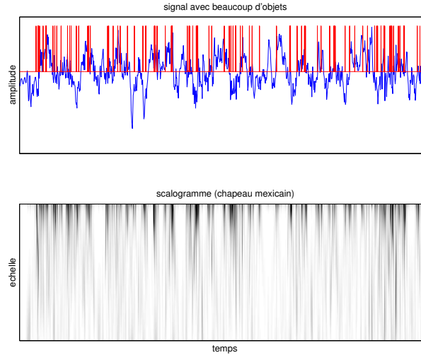
Fig. V.11: Modèle statistique construit sur des objets qui sont des fonctions de Mellin. Sur la trace temporelle du haut on a ajouté des marques positionnant les centres des objets. En dessous la transformée en ondelettes du signal pointe sur certaines singularités mais ne permet pas de retrouver toutes les organisations locales.
