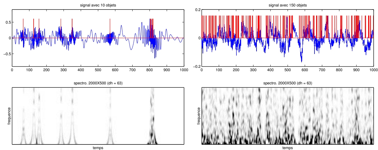
Fig. V.12: Modèle statistique construit sur des fonctions de Mellin, à gauche avec une faible densité d'objets, à droite avec une forte densité. Les positions centrales des fonctions sont indiquées par les barres verticales. Les décompositions temps-fréquence du dessous montrent que seuls les cas avec peu d'objets vont permettre de retrouver les chirps qui ont été mis dans le signal.
