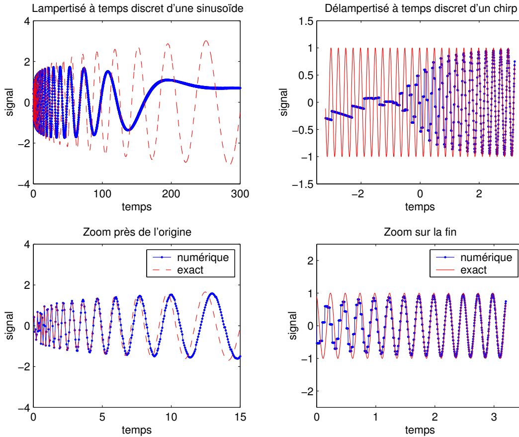
Fig. 11.20: Utilisation de la discrétisation de \mathcal{L}_H selon (II.309) sur une sinusoïde (à gauche) et de \mathcal{L}_H^{-1} sur un chirp (à droite). Bien que la forme est convenable à certains moments (les zooms du bas), le fait que le filtre est une impulsion de Dirac trop large pour être une approximation numérique satisfaisante, amène des mélanges entre les oscillations qui détruisent le résultat petit à petit.
