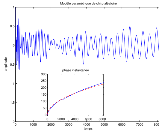
Fig. IV.17: Réalisation d'un chirp aléatoire à phase en \sqrt{t} par contrôle de la position des pôles d'un AR non stationnaire. La phase instantanée mesurée est mise en encart (superposée au comportement théorique attendu). La construction est décrite dans le texte.
