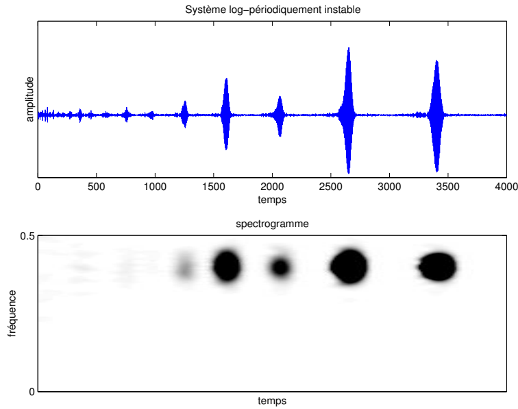
Fig. IV.15: Exemple de sortie d'un EC(2) instable log-périodiquement. Alors que l'allure du processus est proche de la DSI (avec des bouffées d'activité géométriquement espacées), il n'est pas à DSI telle que nous l'étudions ici puisque les statistiques du processus divergent autour des bouffées d'activité. Nous avons obtenu l'exemple en laissant le pôle aller jusqu'à un rayon égal à 1.025. Les périodes d'activité correspondent au moment où le système est instable et s'élargissent car il réside, du fait du ralentissement des oscillations log-périodiques, de plus en plus longtemps dans la zone instable ce qui amplifie son amplitude et demande ensuite plus longtemps à revenir vers les valeurs du système stable.
