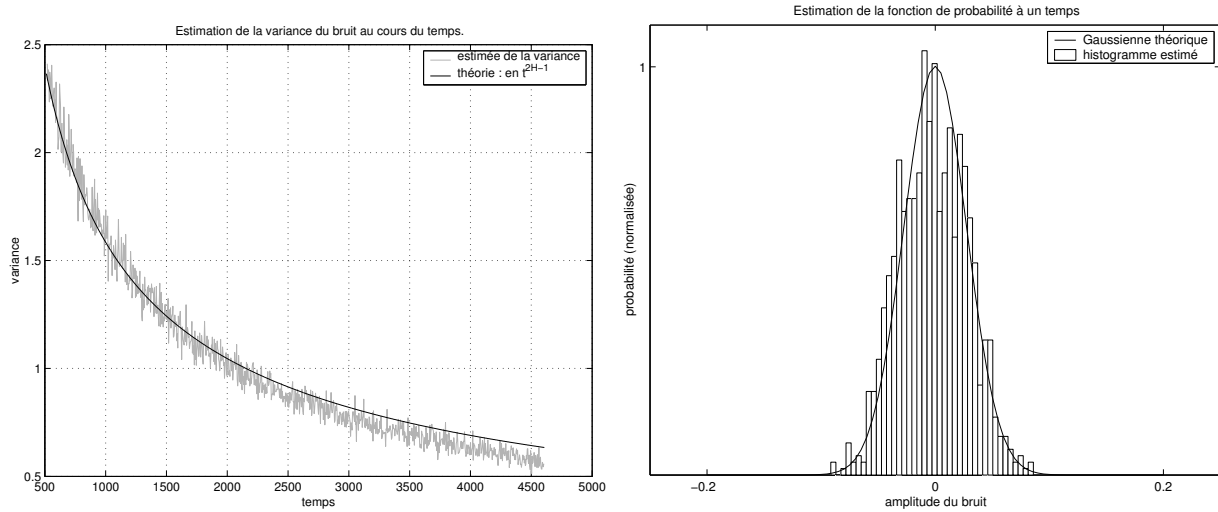
Fig. II.22: Analyse de l'EC d'ordre 1 synthétisé par sa fonction de transfert multiplicative (comme en figure II.21). Nous estimons le bruit du modèle après rééchantillonnage arithmétique comme e_k = X_\tau[k] - a_k X_\tau[k-1] ; les estimations sont faites sur 1000 réalisations. À gauche on montre l'estimation de la variance de ce bruit superposée au modèle (II.318) ; à droite c'est la fonction de probabilité à un temps du bruit représenté comme un histogramme qui est comparée à la loi normale attendue. Nous n'avons pas représenté la corrélation du bruit qui est bien trouvée très courte (bruit quasi blanc). Cette étude valide la synthèse par filtre multiplicatif comme comparable à la discrétisation du modèle par Noret [Nor99].
