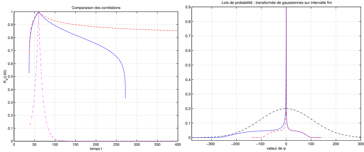
Fig. III.12: À gauche, corrélations des processus OU transformés de la figure III.11 (une borne -- ou deux bornes -), comparées à la corrélation - du processus d'OU initial avec a = 0.2 . À côté, loi de probabilité Gaussienne transformée par (III.178) en une loi sur un intervalle fini. L'intervalle est borné aux deux extrémités et la loi est alors symétrique, tracée en --; l'intervalle n'est borné que d'un seul côté et conduit à la loi non symétrique en -. On a tracé en trait mixte - une gaussienne non bornée pour comparaison.
