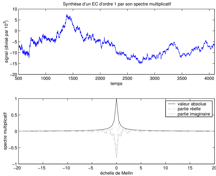
Fig. 11.21: Exemple de synthèse d'un EC d'ordre 1 (en haut) à partir de son spectre multiplicatif (en bas on montre \mathbf{G}_{H,a}(H + i2\pi\beta) déduit de (II.281)) qui est du type passe-bas pour le modèle étudié par Noret. La phase du spectre a été choisie i.i.d. dans [0; 2\pi[ , H = 0.2 et a = 1 . L'échantillonnage résultant de la synthèse est géométrique.
