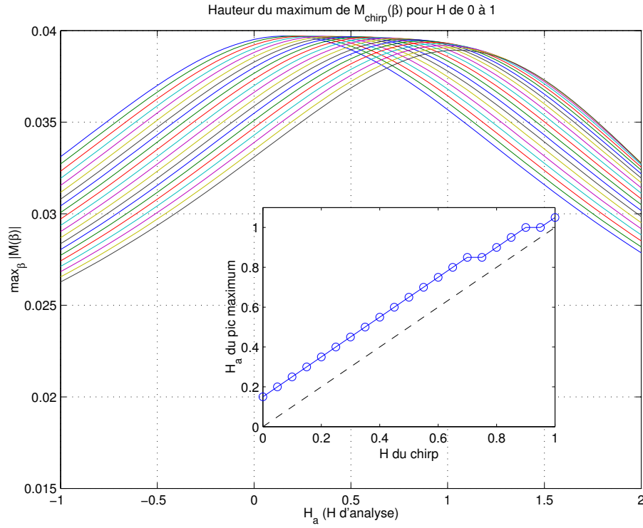
Fig. II.13: Étude de la hauteur du pic maximal pour un chirp H en fonction de H_a d'analyse. Les courbes sont pour H de 0 à 1, se décalant régulièrement vers la droite. L'écart montre la position du maximum pour H en fonction de H_a ; bien que la relation reste globalement linéaire, un biais systématique de 0.2 environ existe.
