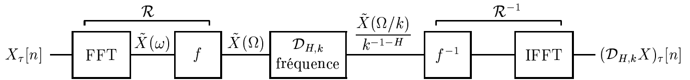
Fig. II.17: Schéma bloc de l'opérateur de dilatation noté \mathcal{D}_{H,k}^{(d)} à temps discret construit sur la transformation bilinéaire [ZR98].
