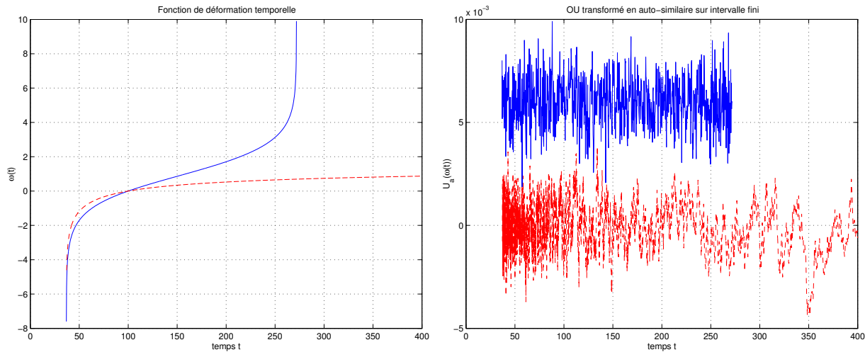
Fig. III.11: À gauche sont tracés les warpings \omega(t) pour une -- et deux -- limites. À côté on montre deux exemples d'un processus OU modifiés en temps par \omega(t) , selon qu'il y a une -- ou deux bornes -- (courbe décalée arbitrairement par une constante).
