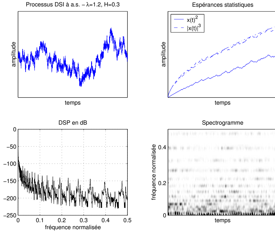
Fig. IV.13: Exemple de réalisation de processus à DSI et accroissements stationnaires à l'aide de la généralisation construite à partir de la fonction de Weierstrass. La synthèse est faite à l'aide de la méthode de la matrice circulante. Paramètres H=0.3 et \lambda = 1.2 . On présente l'estimation des deux premiers moments à droite (avec en traits mixtes le comportement théorique attendu en t^{2H} de la variance); le spectre d'une réalisation en bas à gauche et une représentation temps-fréquence correspondante. Sur les deux, la répartition en série géométrique des principaux modes en fréquence y sont bien visibles.
