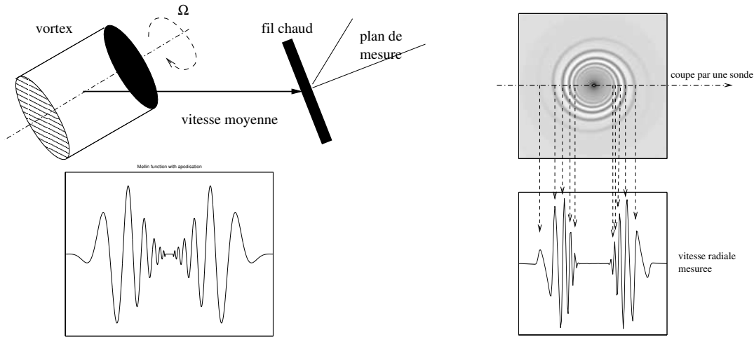
Fig. V.7: L'étude des modèles statistiques d'objet est supposée être à la confrontation des descriptions de vortex (géométriques ou de type dynamique) (en haut), des mesures par des coupes unidimensionnelles qui donnent des fonctions qui ressemblent à des chirps (en bas à droite) et des descriptions mathématiques par des singularités oscillantes qui sont les limites de ces chirps (en bas à gauche, une fonction de Mellin multipliée par une fonction d'apodisation).
