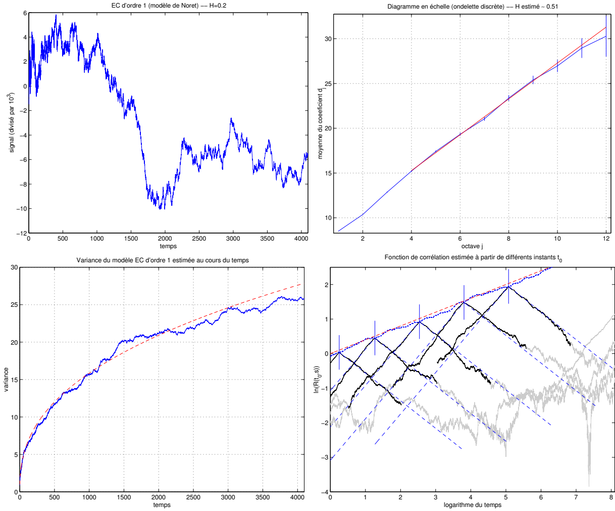
Fig. 11.23: Exemple de réalisation du modèle d'EC d'ordre 1 (en haut à gauche), pour H = 0.2 . Nous montrons, estimée sur 1000 réalisations, la variance du processus (en bas à gauche) et la corrélation (où a contrôle les décroissances en diagramme log-log) (en bas à droite) sur lesquelles les comportements théoriques sont surimprimés en traits pointillés. En haut à droite nous illustrons la non stationnarité importante du modèle : les coefficients d'une décomposition en ondelettes ne sont pas stationnaires (ils croissent en fait tous en t^H ) et l'analyse par diagramme en échelle [AFTV00] conduirait à une mauvaise estimation de H , ici H \simeq 0.51 \pm 0.02 .
