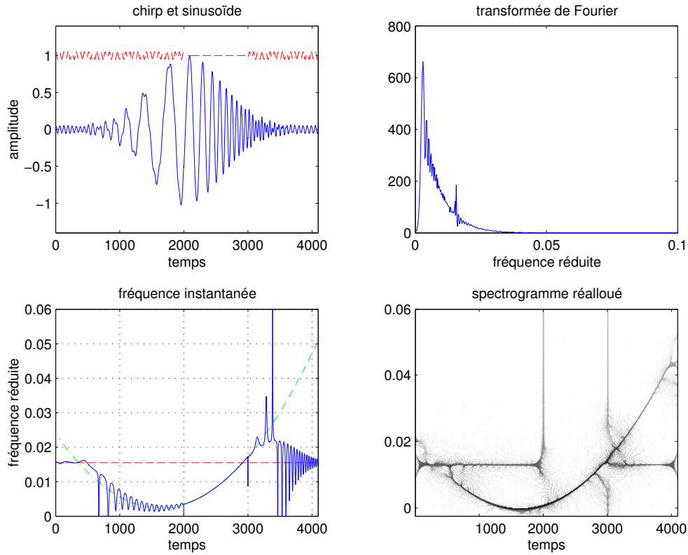
Fig. III.3: Étude d'un signal non stationnaire composé d'un chirp (fréquence instantanée quadratique) superposé à une fréquence pure de faible amplitude qui s'interrompt au milieu. Nous montrons la transformée de Fourier ainsi que la fréquence instantanée qui ne sont pas des descriptions suffisantes pour suivre intuitivement les diverses fréquences du signal. En bas à gauche, la fréquence instantanée donnée par (II.25) est tracée avec celles théoriques des deux composantes du signal : sinusoïde (fréquence constante) et chirp dont la fréquence évolue en temps (ici en parabole). Une représentation temps fréquence, en bas à droite, permet de représenter puis mesurer l'évolution dans le temps du contenu fréquentiel du signal (ici un spectrogramme réalloué - voir [CM98] par exemple).
