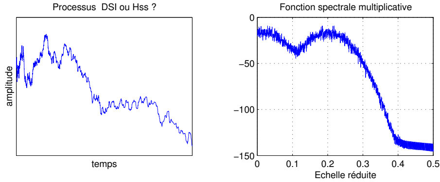
Fig. IV.7: Exemple de processus construit avec des séries de Mellin aléatoires, sous une forme a_1(t)t^{H+i2\pi\beta_1} + a_2(t)t^{H+i2\pi\beta_2} (voir l'équation (IV.29)). À gauche une réalisation du processus, à droite la fonction spectrale multiplicative sur la diagonale. Processus H -ss ou à DSI ? Voir la réponse en figure IV.8.
