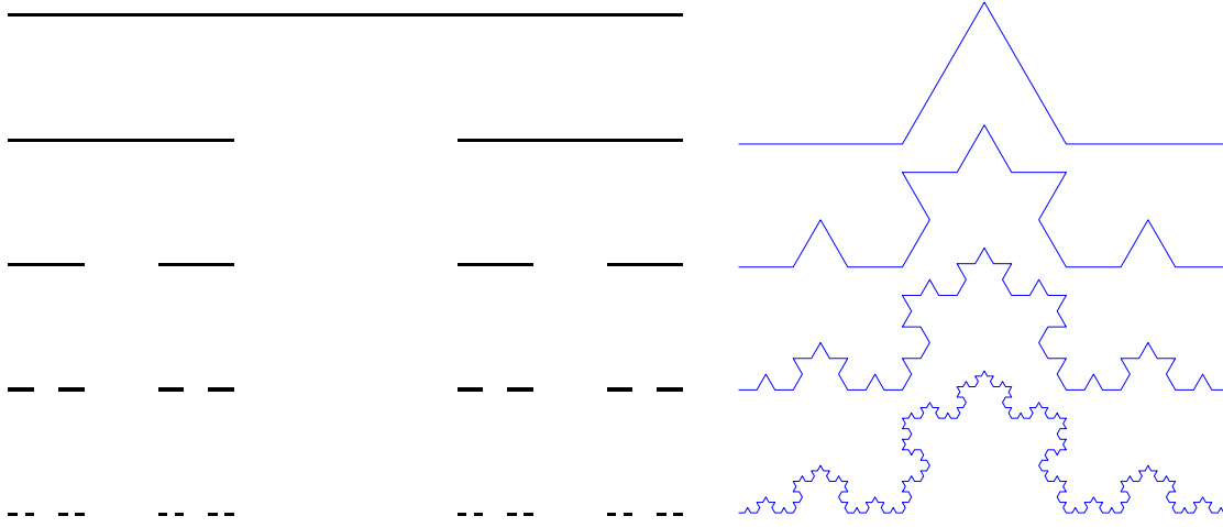
Fig. IV.1: Construction d'un ensemble de Cantor triadique à gauche et d'un côté du flocon de von Koch à droite. Ces deux figures fractales sont bâties sur un rapport d'échelle privilégié de 1/3 et sont alors lacunaires ou à DSI.
