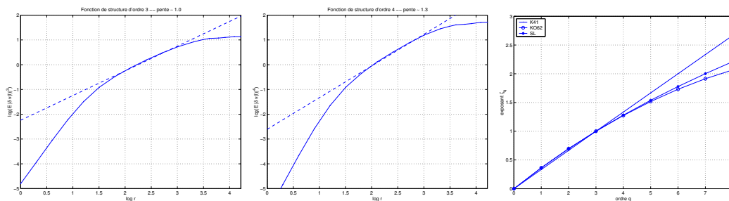
Fig. V.3: Estimations des fonctions de structures S_3(l) (à gauche) et S_4(l) (au centre) et regression linéaire dans la partie correspondant à la zone inertielle. Les lois de puissance sont à l'évidence des approximations seulement dans ce régime, et les exposants sont (au moins sommairement) en accord avec les modèles d'intermittences connus. Le graphe de droite montre les prédictions de différents modèles ; étant proches les unes des autres, elles ne sont pas faciles à discriminer (voir par exemple [Gag87]) – le point durablement établi est que la théorie K41 ne peut tenir et qu'une correction tenant en compte l'intermittence est nécessaire.
