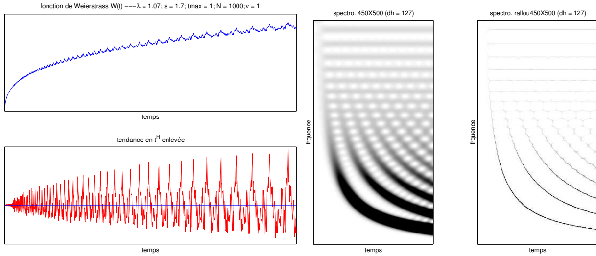
Fig. IV.11: À gauche on a tracé une fonction de Weierstrass déterministe et la même fonction une fois le mode de croissance général en t^H enlevé (il ne reste que les oscillations de la DSI). À droite se trouvent les décompositions temps-fréquence (spectrogramme et spectrogramme réalloué) où sont bien visibles la double lecture possible pour W(t) : une somme de chirps hyperboliques (détectés à basse fréquence quand la fenêtre du spectrogramme est de largeur comparable à la période au plus des fréquences cherchées) ou une somme de modes géométriquement espacés en fréquence (détectés quand la fenêtre est grande devant les périodes testées).
