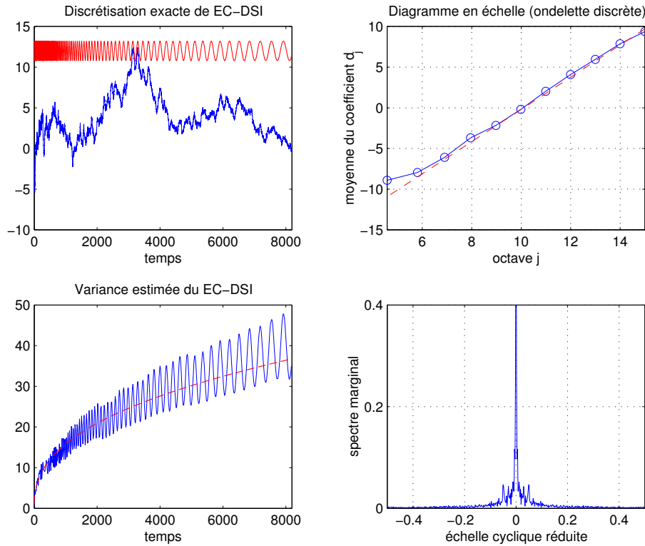
Fig. IV.14: Exemple de réalisation d'un processus d'Euler-Cauchy d'ordre 1 à DSI; H = 0.2 , \lambda = 1.05 . On a superposé au graphe du processus une évolution synchronisée avec le coefficient log-périodique pour référence. En haut à droite on montre le diagramme en échelle qui ici a une pente conduisant à une fausse estimation de H comme 0.5 (processus dont les accroissements ne sont pas stationnaires). En bas, nous montrons la DSI à l'aide d'une part de l'évolution de la variance du processus au cours du temps, d'autre part du résultat d'estimation du spectre marginal cyclique sur une réalisation. Les deux pics de part et d'autre du pic central sont bien à la fréquence correspondant à la log-période, mais restent ici peu visibles.
