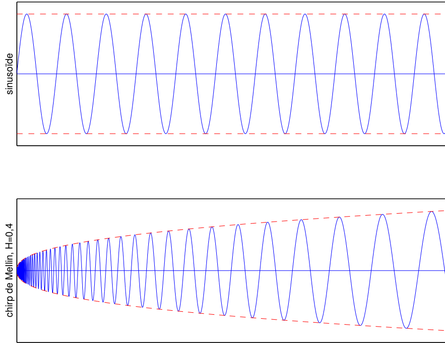
Fig. II.4: La transformée de Lamperti de la sinusoïde, qui réside à une fréquence unique, est un chirp de Mellin (représenté en-dessous) dont l'amplitude croît en t^H et la phase est modulée logarithmiquement.
