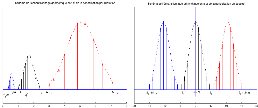
Fig. II.10: Schématisation de l'échantillonnage conjoint en temps (à gauche) et en échelle de Mellin (à droite) qui indique les périodisations induites.
