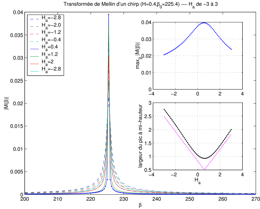
Fig. II.12: Transformation de Mellin discrète d'un chirp E_\beta^H(t) ; l'indice d'amplitude H_a pour la TMD varie de -3 à 3. On a tracé en encart la hauteur des pics et en-dessous leur largeur à mi-hauteur (les points sont le calcul numérique comparé à la variation en - que prévoit le calcul analytique du texte). Remarquons que le pic s'élargit et diminue quand on s'éloigne du H_a = H + 0.2 .
