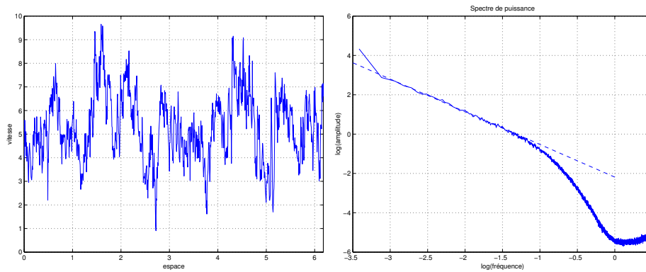
Fig. V.1: Extrait d'un signal de vitesse de turbulence, rééchantillonné en espace par hypothèse de Taylor locale. Les signaux viennent des expériences de C. Baudet et A. Naert (ENS Lyon). À droite, spectre de vitesse estimé par périodogramme. La régression linéaire dans la zone inertielle est en accord raisonnable avec (V.13) et a une pente proche de -5/3 .
