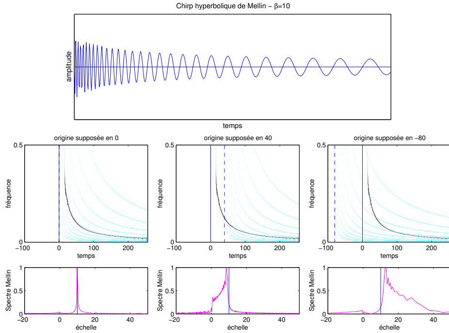
Fig. II.15: Interprétation tomographique de la transformation de Mellin et de l'erreur due à une origine incertaine. Le signal est représenté en haut, et sa décomposition en temps t et fréquence f (spectrogramme réassigné) est indiquée en dessous. De gauche à droite on montre les cas où l'origine supposée pour l'analyse est correcte (trait plein), trop à droite ( t_0 = 40 ) ou trop à gauche ( t_0 = -80 ) (l'origine pour l'analyse est le trait pointillés). En pointillés et en gris sont tracées les hyperboles d'analyse qui croisent plus ou moins l'hyperbole en noir qui est la trace en (t, f) du signal. Le fait que la signature est tronquée (ici par exemple vers f \simeq 0.25 près de l'origine des temps) explique que la bande spectrale de la TMD estimée est aussi limitée quand l'origine est fausse. Sur les transformée de Mellin du bas, on a indiqué d'un trait la position de l'échelle de Mellin réelle du chirp.
