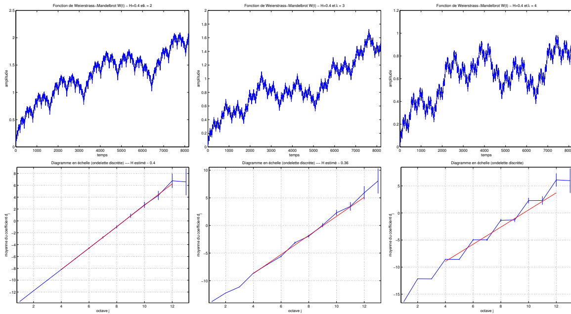
Fig. IV.12: Trois exemples de fonctions W(t) pour H = 0.4 avec \lambda égal à 2, 3 et 4 de gauche à droite. En-dessous on a calculé la représentation en ondelettes moyennée sur le temps comme en (IV.45) et tracée en log-log. Selon la valeur de \lambda par rapport au pas d'analyse (ici sur la grille dyadique qui privilégie les rapports d'échelle de valeur 2), soit on ne voit pas la DSI ( \lambda = 2 ), soit elle est flagrante (si \lambda = 4 ) soit, et c'est le cas général, elle perturbe l'estimation de H du fait des légères oscillations sans donner lieu à une fréquence en échelle facilement identifiable sur ce diagramme en échelle (ici cas où \lambda = 3 ).
