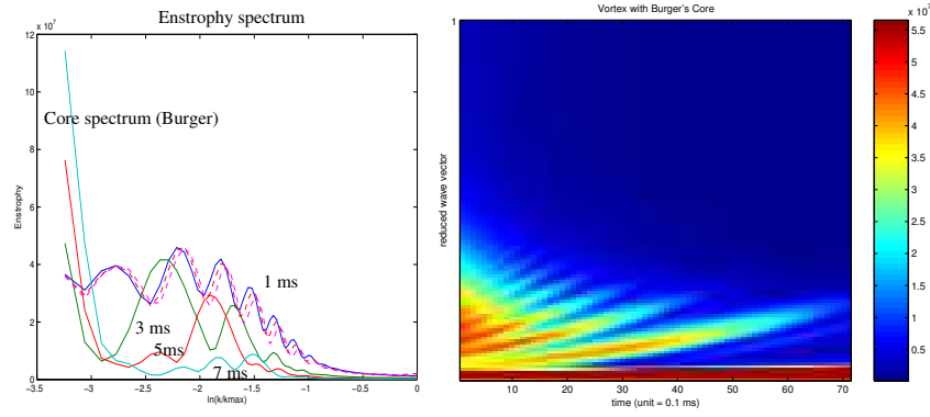
Fig. V.14: Évolution instantanée de l'enstrophie d'un vortex de la classe de Lundgren, à cœur en vortex de Burgers \omega_0(r) \propto (1+hr^2)e^{-r^2} . On notera que le spectre d'enstrophie semble au cours du temps se répartir sur des bras qui migrent vers les petites échelles (de Fourier).
