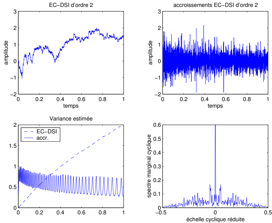
Fig. IV.16: Exemple de réalisation d'un processus d'Euler-Cauchy d'ordre 2 à DSI ; H = 0.3 , \lambda = 1.05 . On montre une réalisation du processus à gauche et de ses accroissements à droite. En dessous, une analyse numérique est conduite en deux étapes. À gauche l'estimation de la variance du processus en révèle la croissance générale (en t^{2H} ) tandis que la variance des accroissements est plus sensible à l'invariance en échelle discrète que vérifie le processus. À droite l'estimation du spectre marginal cyclique sur une réalisation du processus confirme la propriété de DSI pour ce modèle.
