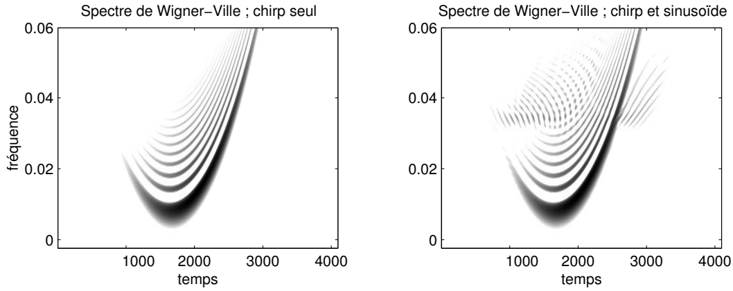
Fig. III.4: Distribution de Wigner-Ville du même chirp que pour la figure III.3 à gauche, et de l'addition de ce chirp et de la sinusoïde (interrompue au centre) à droite. On note combien les oscillations que causent les interférences internes au signal compliquent la lecture pratique de la distribution temps-fréquence. En particulier la composante de fréquence constante (figure de droite) est cachée dans les oscillations.
