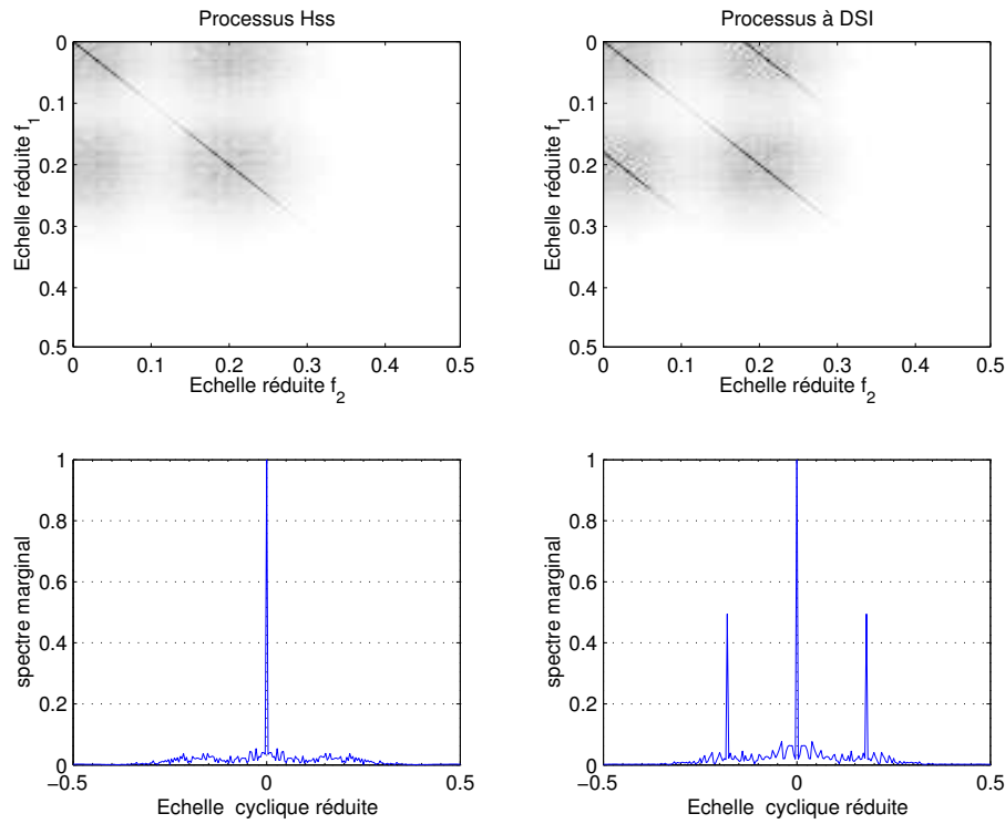
Fig. IV.8: Le processus précédent de la figure IV.7 peut être au choix synthétisé avec des propriétés auto-similaires (si \mathbb{E}\{a_1(t)\bar{a}_2(t)\} = 0 ) ou de DSI sinon. Alors que le spectre multiplicatif moyen est le même, l'estimation de la fonction spectrale multiplicative (en haut) puis du spectre marginal en échelle cyclique révèlent l'auto-similarité du premier cas et l'invariance en échelle discrète dans le second dont on estime le facteur en échelle privilégié à l'aide des pics de part et d'autre du pic central dans le spectre marginal cyclique..
