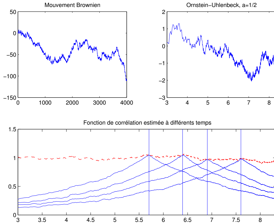
Fig. II.5: Transformée de Lamperti pour un processus d'OU, a = 1/2 . On montre en dessous le comportement estimé numériquement de la corrélation de (\mathcal{L}_{1/2}^{-1}B)(t) à partir de certains instants : la décroissance est bien exponentielle. La ligne en pointillés est l'estimation de la variance au cours du temps (stationnaire). Les estimations sont des moyennes d'ensemble sur 10^3 réalisations.
