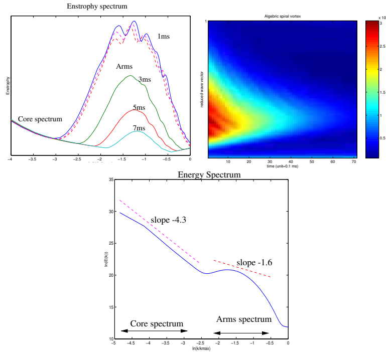
Fig. V.17: Évolution instantanée de l'entrophie d'un vortex de la classe de Lundgren, dont l'enroulement est en spirale algébrique, \Omega(r) \propto r^{-\alpha} .
