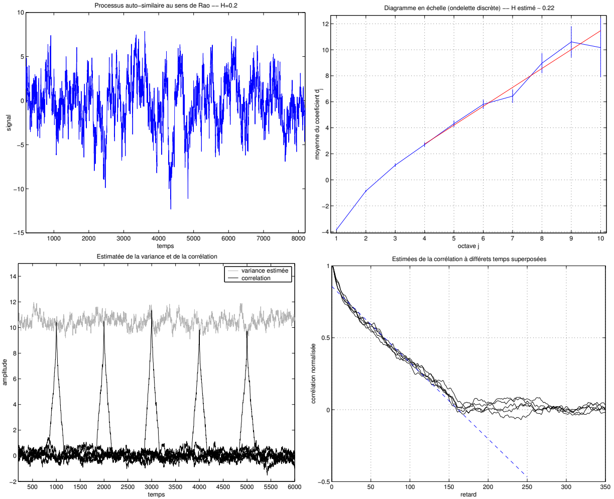
Fig. 11.24: Exemple de réalisation du modèle H -ss de Rao (en haut à gauche), pour H = 0.2 . Nous montrons, estimée sur 1000 réalisations, la variance au cours du temps et la fonction de corrélation à certains instants (en bas à gauche). La variance reste constante et les fonctions de corrélations, superposées sur le graphe adjacent, sont identiques à tout instant : le processus est stationnaire. Cependant il est approximativement H -ss par ses propriétés de régularité locale en temps et l'analyse par une décomposition en ondelettes (en haut à droite) conduit à estimer correctement l'exposant H de la séquence synthétisée, ici H \simeq 0.22 \pm 0.05 .
