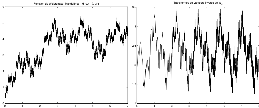
Fig. IV.2: Délampertisation d'un processus à DSI, ici une fonction de Weierstrass (voir 2.5 pour sa définition). La fonction originelle est à gauche et est log-périodique, son image par \mathcal{L}_H^{-1} est à droite et est périodique dans le temps.
