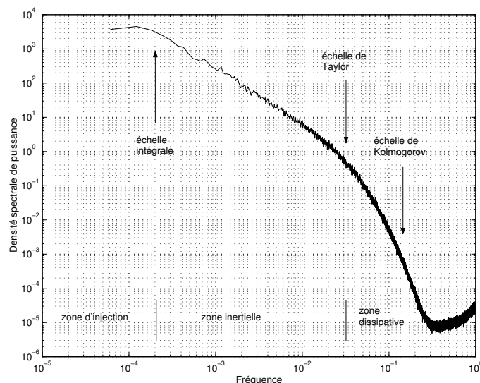
Fig. III.7: Spectre typique du signal de vitesse d'un jet turbulent. Données des expériences de C. Baudet et A. Naert (ÉNS Lyon) [BMW99]. L'existence d'une grande échelle (échelle intégrale) et d'une coupure à petite échelle (échelle visqueuse ou de Kolmogorov) est un ingrédient de base des propriétés en échelle de la turbulence (voir le chapitre V pour une présentation du problème).
