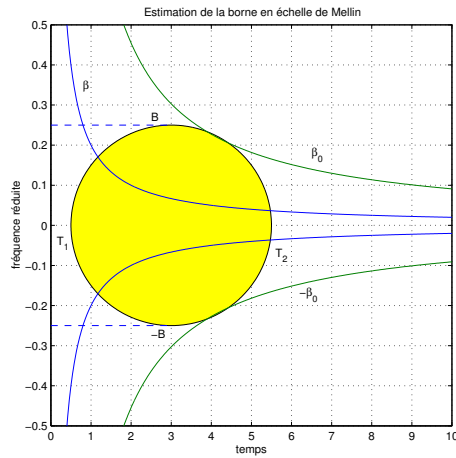
Fig. II.11: Estimation dans le plan temps-fréquence de l'extension en échelle de Mellin d'un signal.
