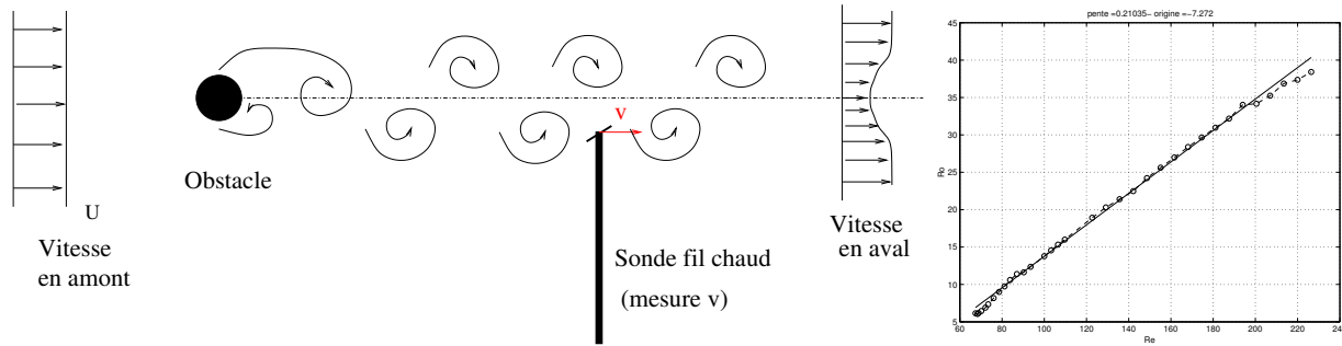
Fig. V.4: Sch matisation de l'all e de vortex altern s de von K rm n [Wil96] que nous avons  tudi e. Nous reportons   droite la caract ristique mesur e du nombre de Reynolds Re = Ud/\nu en fonction du nombre de Roshko Ro = fd^2/\nu . \nu est la viscosit , d = 3 mm le diam tre du barreau, et f est la fr quence fondamentale des oscillations du sillage. L'accord avec la relation de Roshko, Ro = 0.212 Re - 4.5 est acceptable.
