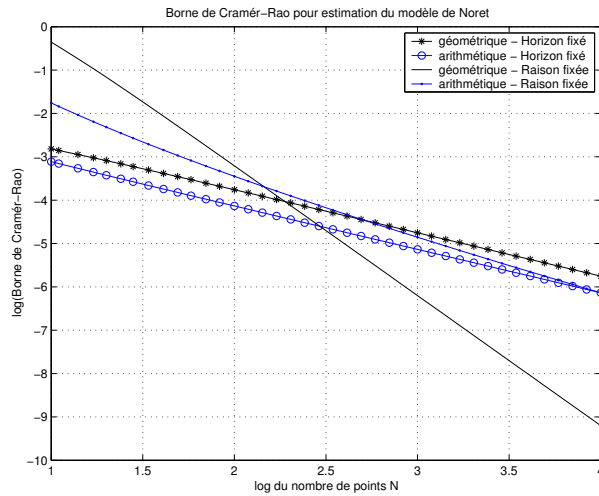
Fig. 11.16: Évolution de la borne de Cramér-Rao pour l'estimation de H du modèle X_{H,a} de Noret [NG99]. Les échantillonnages géométriques et arithmétiques sont comparés. Si l'horizon d'observation est imposé, le deuxième est meilleur ; si c'est la raison de la série, le premier est plus efficace en général (quand l'horizon d'observation devient suffisamment plus grand que celui que donne l'échantillonnage arithmétique). L'horizon d'observation fixé est L = 10^4 .
