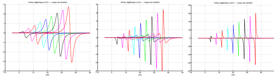
Fig. V.8: Graphe des noyaux de transfert en échelle. À gauche n'est représentée que la fraction \frac{n(2\pi\gamma+2\pi\beta-2i)}{(2-i2\pi(\beta-\gamma))^2} , tandis qu'à droite on a pris Z_0(\beta) = (1 + ih\pi\beta)\Gamma(i\pi\beta)/2 . Sur ce deuxième graphe on montre les cas pour \beta = n2\pi avec n allant de 1 à 3. On constate que le transfert est principalement local (autour de \beta = 0 sur la graphe de gauche et de \gamma = \beta à droite) en échelle.
