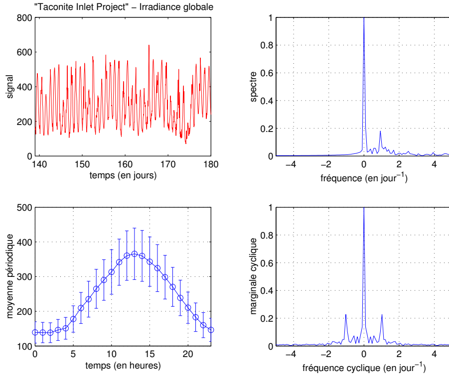
Fig. IV.6: Analyse de l'irradiance globale de la station Delta. Nous montrons en haut à droite le spectre du signal analytique ; en bas à gauche la moyenne périodique empirique de la série de période 24 heures. Elle révèle l'évolution sur la période cyclique des statistiques de la série. Les barres représentent l'estimation empirique de la variance périodique de la série et elle évolue aussi sur 24 h. Enfin la marginale cyclique calculée comme \int_{-\infty}^{+\infty} S^{\nu_c}(v, f)df (voir aussi (IV.27)) est représentée en bas à droite et, en plus du pic central qui est l'énergie du signal, présente les pics symétriques à la fréquence cyclostationnaire.
