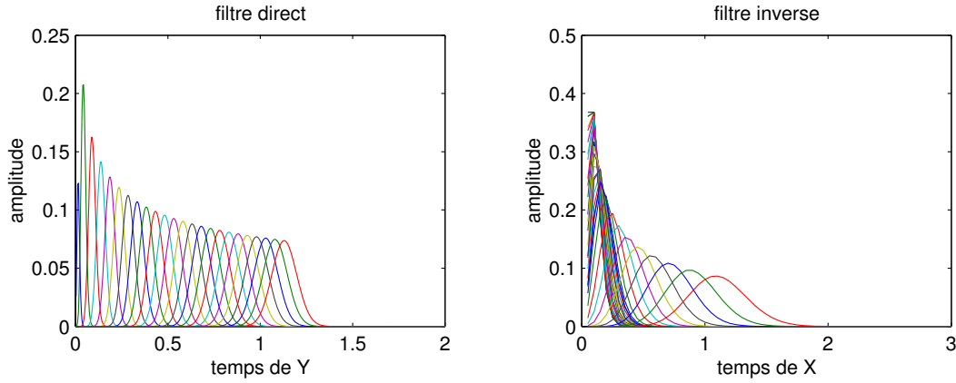
Fig. II.19: Filtres de Lamperti direct et inverse calculés par l'équivalence imposée entre 1 - \mathbf{B} et d/dt selon (II.309). Ces deux filtres sont de mauvaises approximations de pics de Dirac qui se décalent en temps comme t - \ln t et e^t - t .
