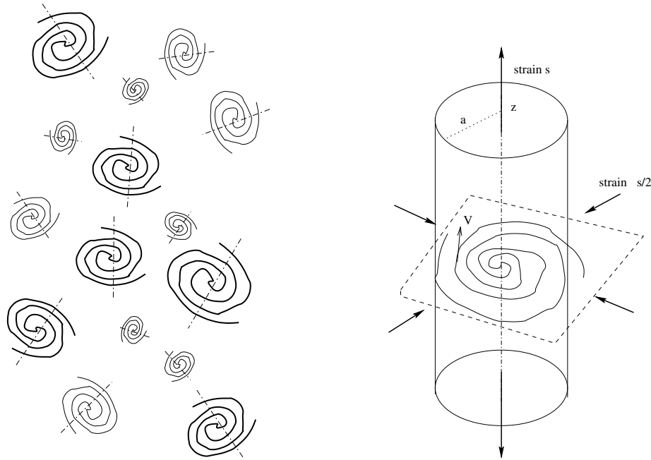
Fig. V.6: Figuration d'un ensemble statistique d'objets structurés ; c'est l'image intuitive du modèle que nous voulons étudier. Les objets sont à structure interne riche, vivent à toutes les échelles, sont instationnaires et ne se mélangent pas. À droite on a représenté le cadre que décrit la solution de Lundgren : un vortex spiralé, étiré selon un axe et dont l'évolution est quasi bidimensionnelle autrement.
