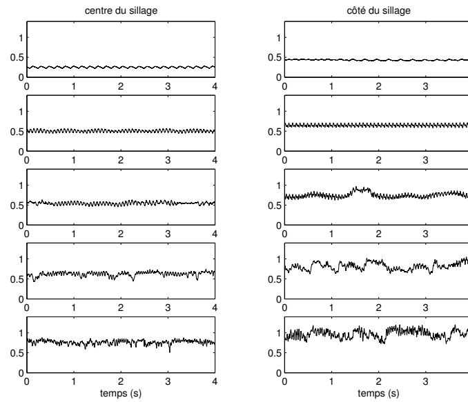
Fig. V.5: Exemples de profils de vitesse (en m/s) dans le sillage quand on augmente la vitesse moyenne en aval du barreau. Ici le Re passe par les valeurs 80, 120, 135, 155 et 190. Les courbes à gauche sont la vitesse au milieu du sillage à 6 cm en aval de l'obstacle de 3 mm de diamètre, à droite le fil chaud a été déplacé perpendiculairement de 1 cm par rapport au centre.
