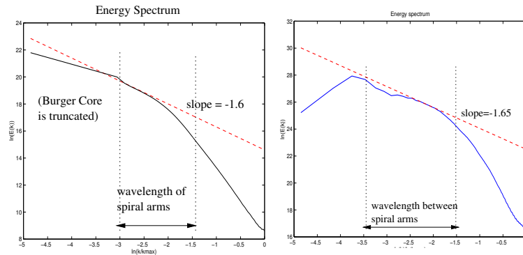
Fig. V.16: Spectre d'énergie moyenné dans le temps, à gauche pour le modèle de la figure V.14, à droite pour celui de V.15
