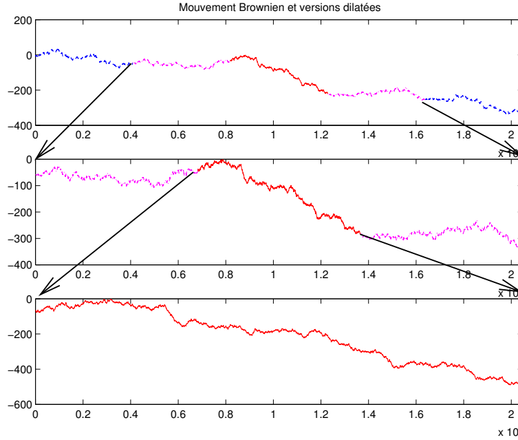
Fig. II.1: Exemple de réalisation d'un mouvement Brownien où l'on a dilaté les parties centrales pour illustrer son auto-similarité.
