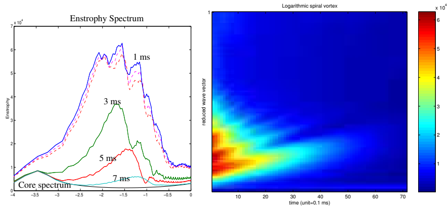
Fig. V.15: Évolution instantanée de l'enstrophie d'un vortex de la classe de Lundgren, dont l'enroulement est en spirale logarithmique ( \Omega(r) \propto (\ln r)e^{-r^2} ).
