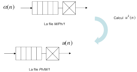
Fig. 4 - Itérations entre les files M/Ph/1 et Ph/M/1.
