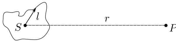
FIGURE 2 – Distribution quelconque de masse : on effectue un développement multipolaire pour r \gg l .
