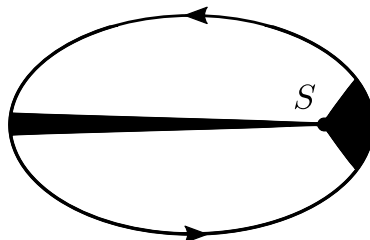
FIGURE 1 – Représentation schématique d'une vitesse aréolaire constante sur une orbite elliptique.
