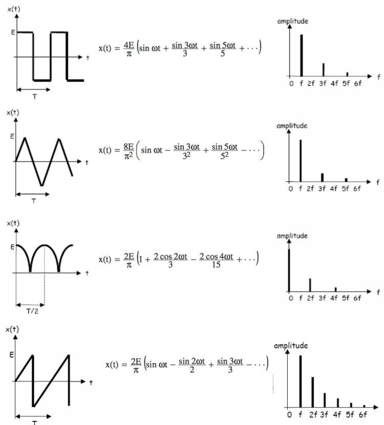
Fig. 1 : Signaux usuels et leur spectre
