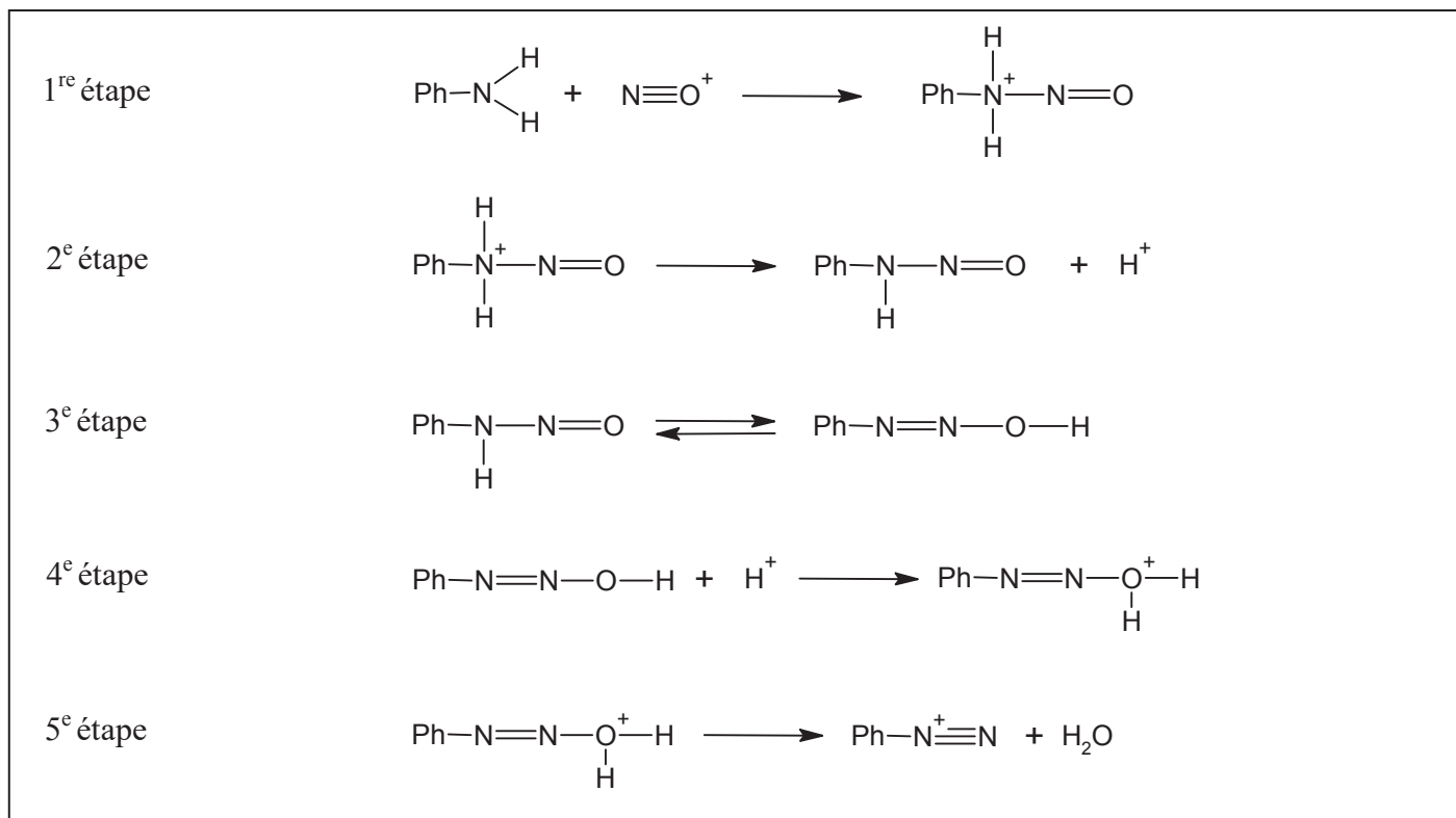
Figure 5 : Mécanisme de formation de l'ion benzènediazonium \text{C}_6\text{H}_5\text{-N}_2^+ par action de l'ion nitrosonium \text{NO}^+ sur l'aniline
