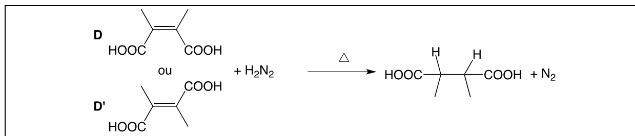
Figure 5 : Hydrogénation par le diimide
