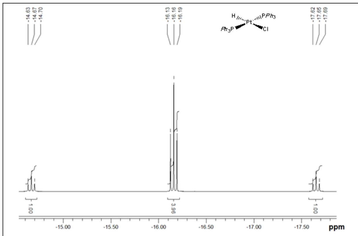
Figure 6 : Signaux obtenus pour l'hydrogène lié au platine dans le spectre RMN ^1\text{H} du complexe [\text{Pt}(\text{H})(\text{Cl})(\text{PPh}_3)_2] (les déplacements chimiques des différents signaux sont pointés en haut du spectre et les valeurs indiquées en dessous des signaux correspondent à leur intégration relative)
