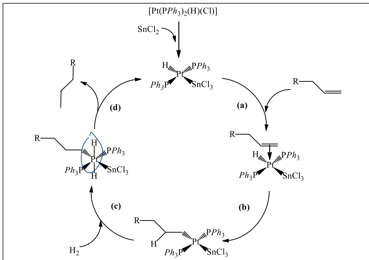
Figure 7 : Cycle catalytique de l'hydrogénation d'un alcène
