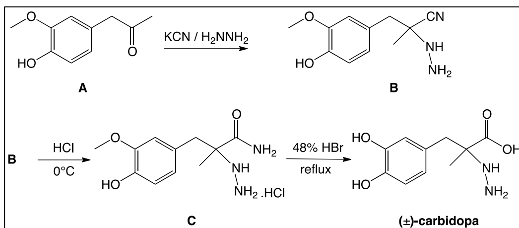
Figure 4 : Voie de synthèse de la carbidopa
