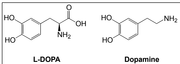
Figure 3 : Structure de la L-Dopa et de la dopamine
