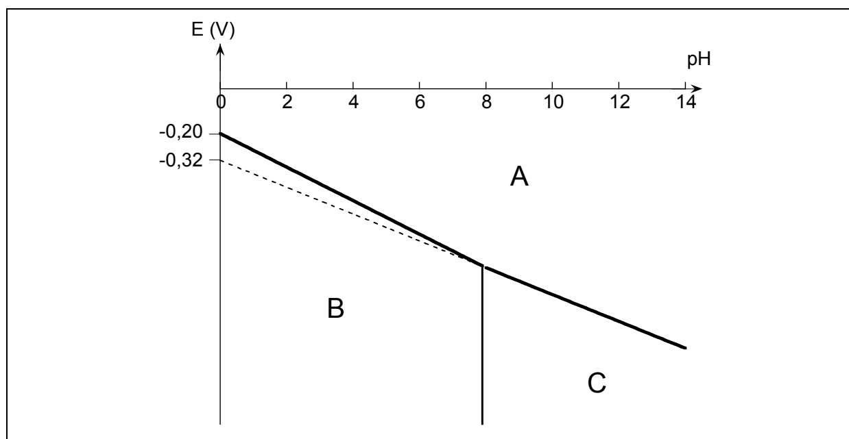
Figure 2 : Diagramme potentiel-pH
