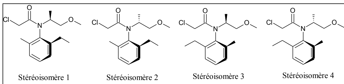
Figure 12 : Stéréoisomères du métolachlore
