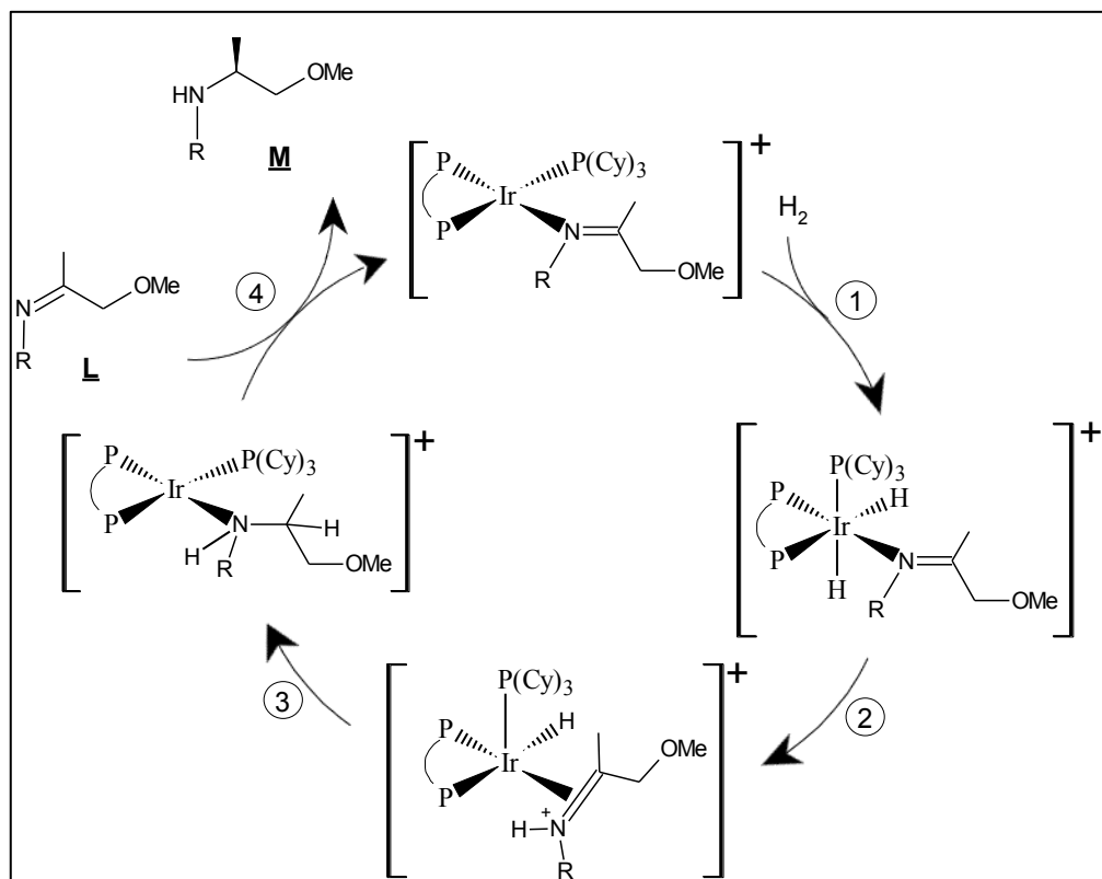
Figure 17 : Cycle catalytique pour l'étape L → M
