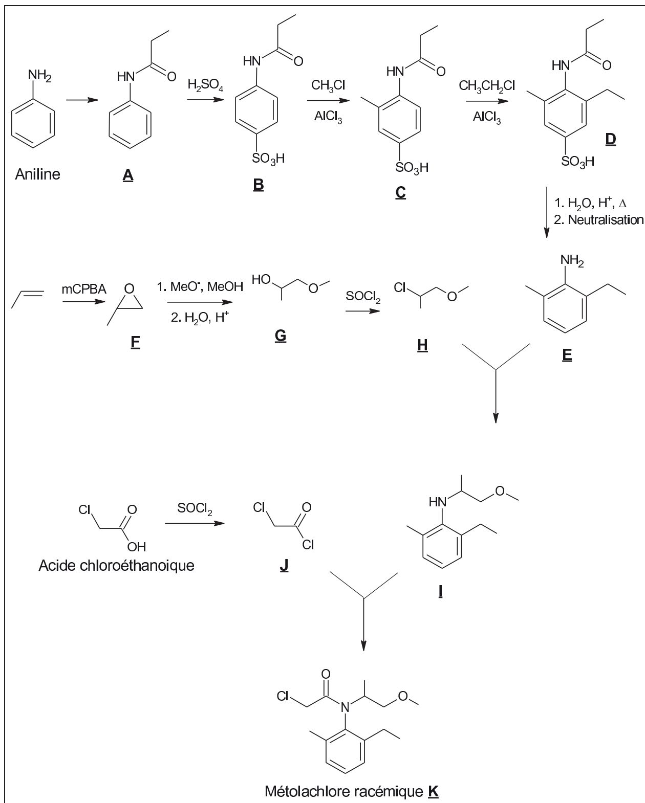
Figure 13 : Schéma de synthèse du métolachlore racémique à partir de l'aniline
