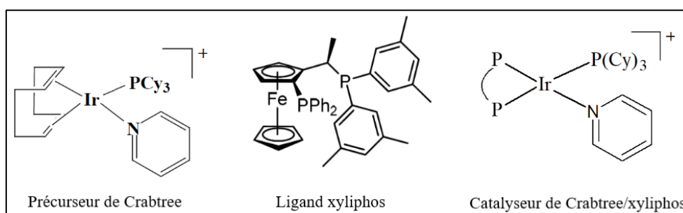
Figure 16 : Catalyseur de Crabtree/Xyliphos. Les notations Cy et Ph désignent respectivement les groupements cyclohexyle et phényle.
