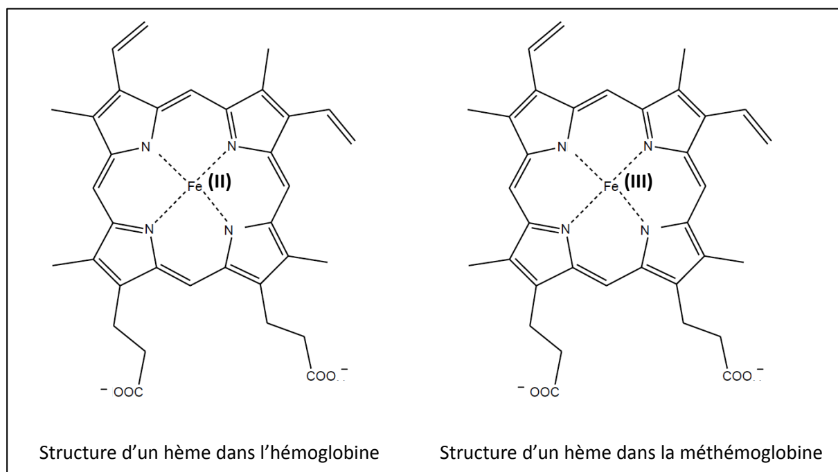
Figure 6 : Structures des hèmes dans les protéines d'hémoglobine et de méthémoglobine
