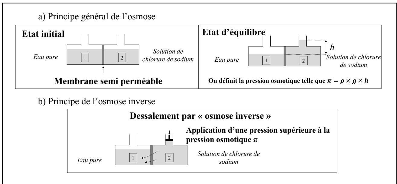
Figure 1 : Principe de l'osmose (a) et de l'osmose inverse (b) 1
