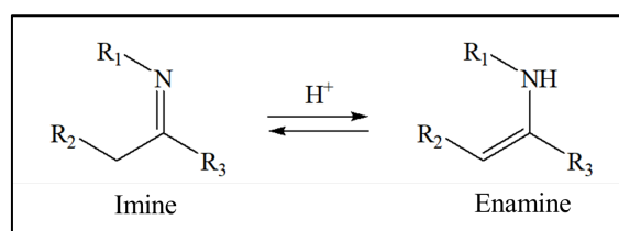
Figure 8 : Équilibre de tautomérie imine – énamine
