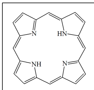
Figure 7 : Structure de la porphine
