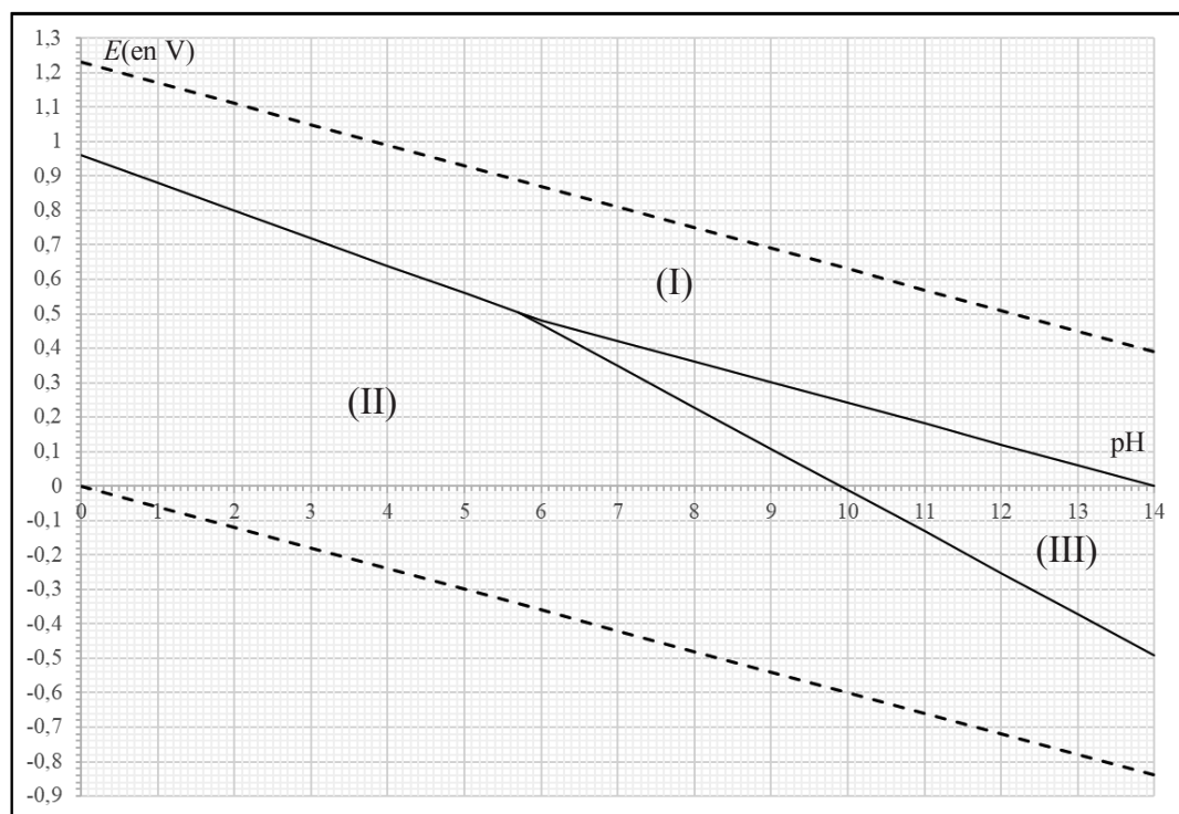
Figure 3 : Diagramme E – pH simplifié de l'élément azote. Les droites en pointillés correspondent au domaine de stabilité thermodynamique de l'eau.
