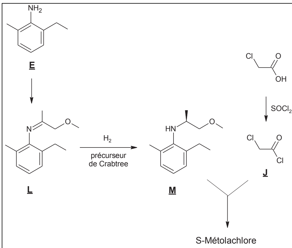
Figure 15 : Schéma de synthèse énantiosélective du S-métolachlore à partir de l'éthylméthylaniline
