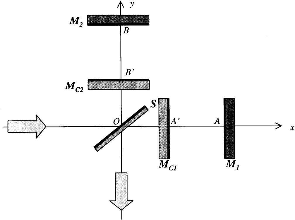
Figure 5 Interféromètre DIOG
