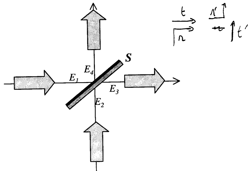
Figure 3 Lame séparatrice
