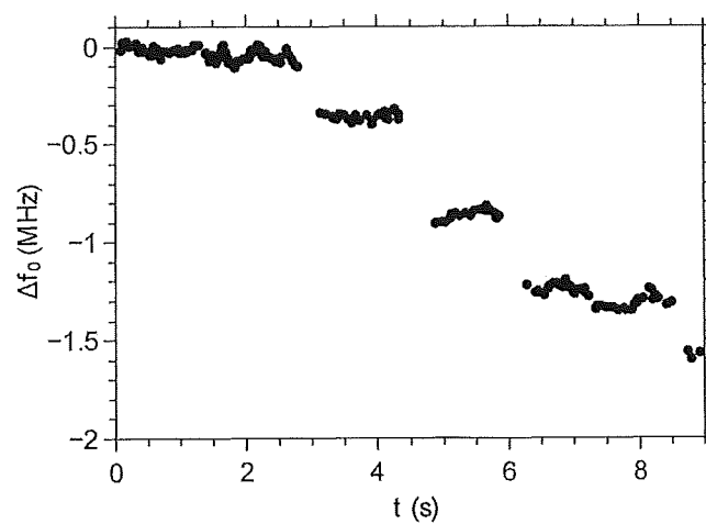
FIGURE 13 – Décalage en fréquence d'un nano-oscillateur de longueur L = 150 nm à 4 K exposé à une faible pression de naphtalène. (D'après J. Chaste et al. , Nature Nanotechnology 7, 301 (2012))
