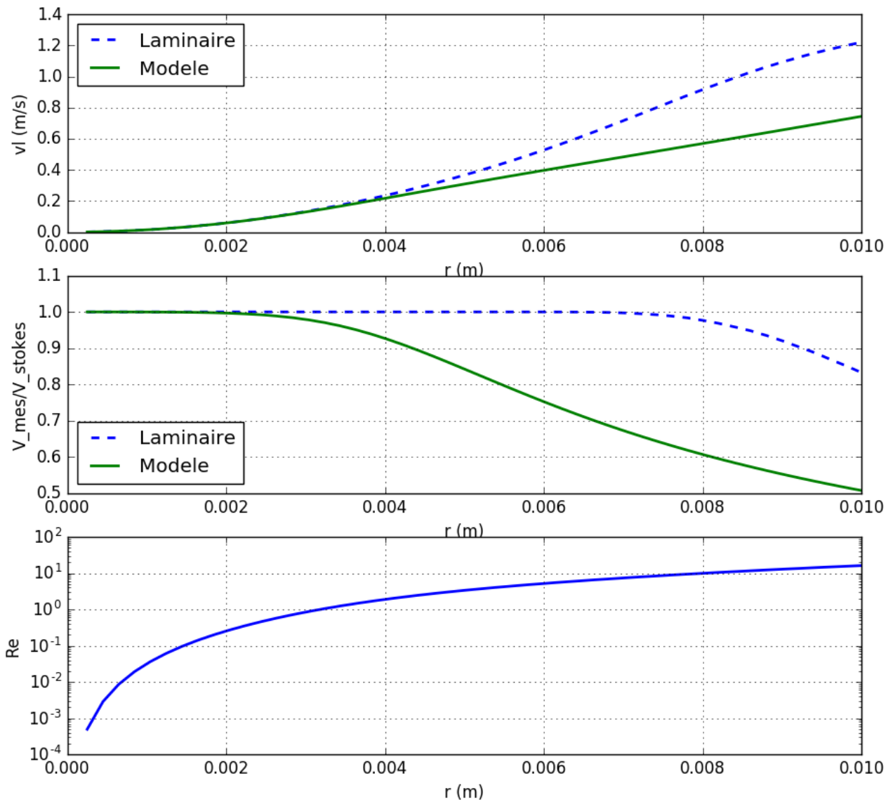
Fig. 4. Résultat du calcul numérique correspondant au code Python 3.5 situé page 27. Les paramètres expérimentaux utilisés correspondent à du glycérol pur à 20°C, et une distance \Delta z = 40\text{cm} .
