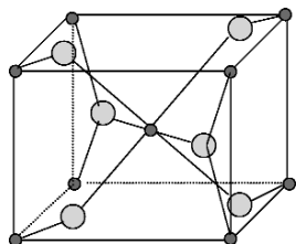
Figure 3 : Représentation de la structure du rutile, \text{TiO}_2 . Les gros cercles représentent les anions oxyde \text{O}^{2-} et les petits les cations titane \text{Ti}^{4+} . La figure met en évidence l'environnement octaédrique du titane. On dénombre 1 + 8/8 = 2 cations titane et 4/2 + 2 = 4 anions oxyde par maille, soit un rapport stoechiométrique en accord avec la formule du rutile.
