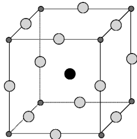
Figure 4 : Structure pérovskite : cas de \text{CaTiO}_3 . L'ion \text{Ca}^{2+} au centre du cube, de rayon voisin de celui de l'ion oxyde est dans un environnement dodécaédrique. L'environnement du titane, au sommet du cube est octaédrique, comme dans le rutile.
