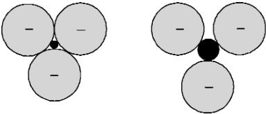
Figure 2 : Représentation à deux dimensions d'un site cristallographique constitué de trois anions dans lequel se loge un cation. À gauche, le rayon du cation est trop petit, les anions se touchent, la répulsion électrostatique est forte. La structure n'est pas stable. À droite, le rayon du cation permet aux anions de ne pas être au contact. La structure est plus stable.
