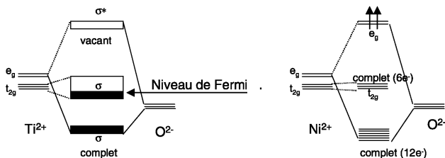
Figure 6 : Représentation des niveaux d'énergie du cristal \text{TiO} (à gauche) et \text{NiO} (à droite).
