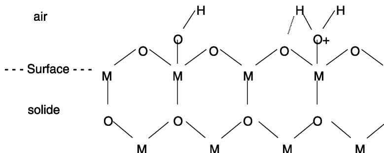
Figure 5 : Représentation de la surface chargée positivement d'un oxyde.
