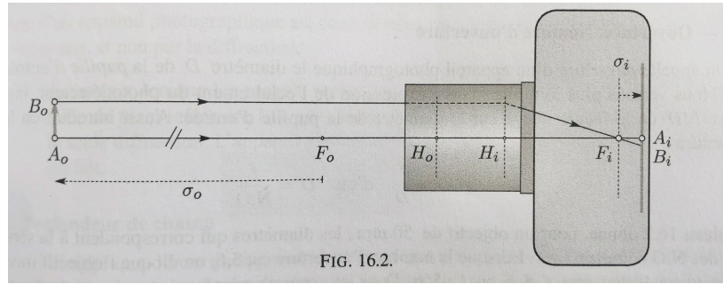
FIGURE 3 – Source : Pérez. À refaire au tableau ou sur inkscape avec une image à distance finie et en confondant les deux centres optiques
