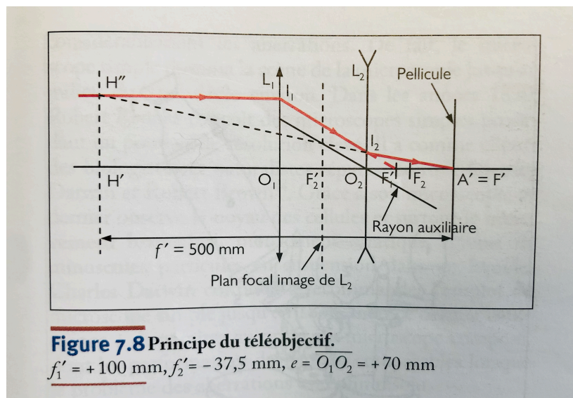
FIGURE 4 – Source : Pérez. À refaire au tableau ou sur inkscape avec une image à distance finie et en confondant les deux centres optiques
