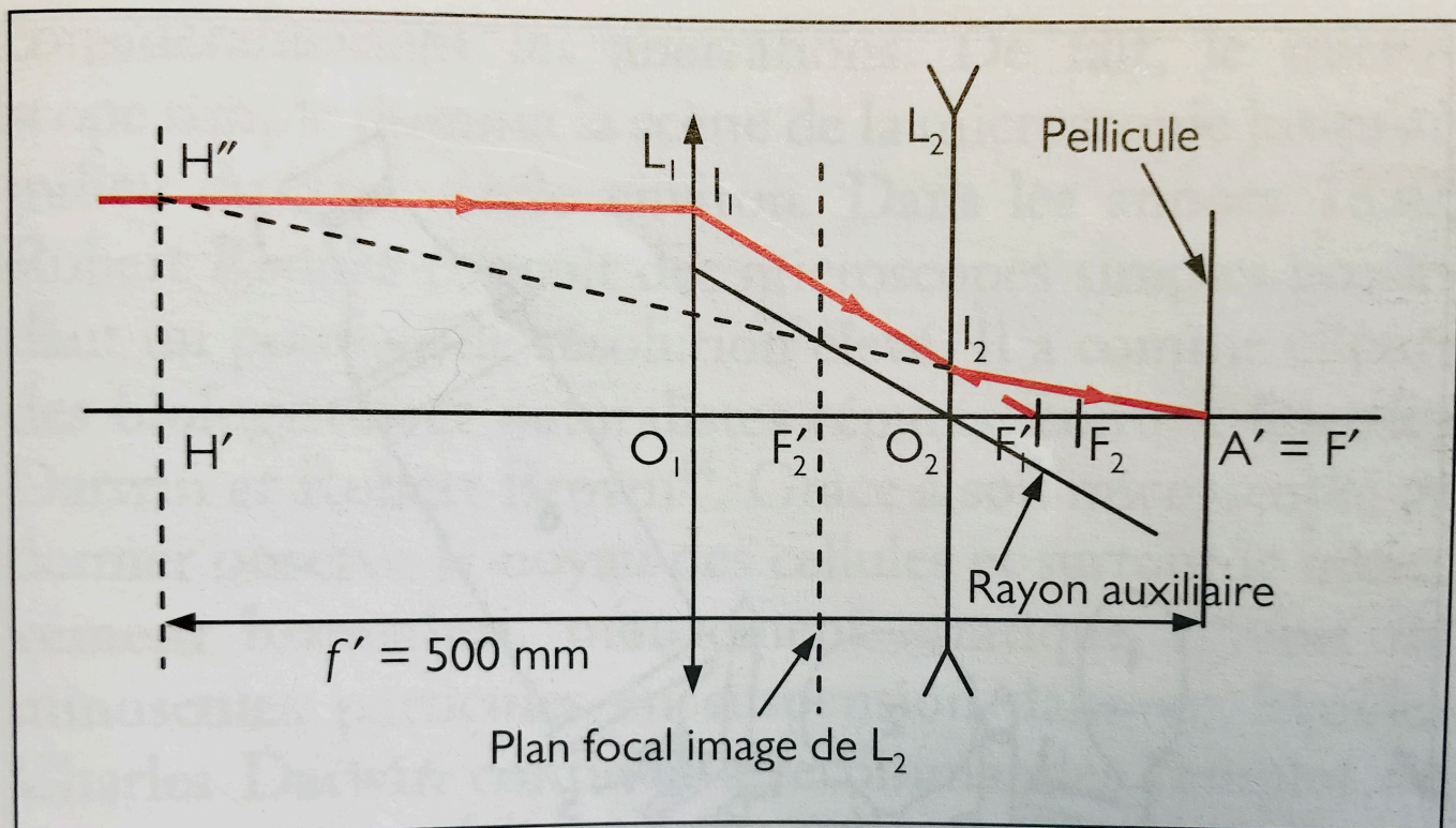
Figure 7.8 Principe du téléobjectif.
