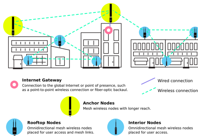
Figure 30. Schéma explicatif du système Mesh =@newamerica.
