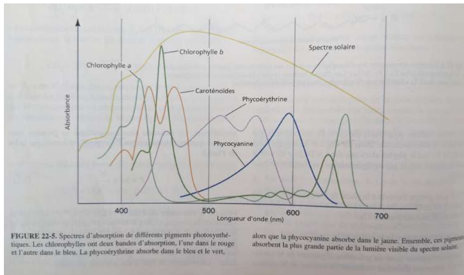
FIGURE 7 – Absorption (Voet)
