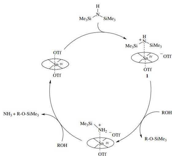
Fig. 7 Cycle catalytique proposé pour un catalyseur à base d'étain utilisé pour réaliser une étape de silylation de surface [27].
