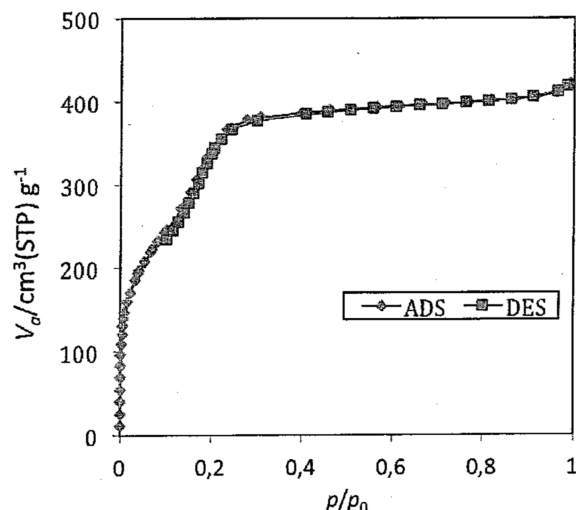
Fig. 14 Isothermes d'adsorption de N_2 à 77 K de la silice calcinée ( S_{BET} = 1060 \text{ m}^2/\text{g} , C = 80 , V_{meso} = 0,60 \text{ cm}^3/\text{g} , dp = 2,0 \text{ nm} ).
