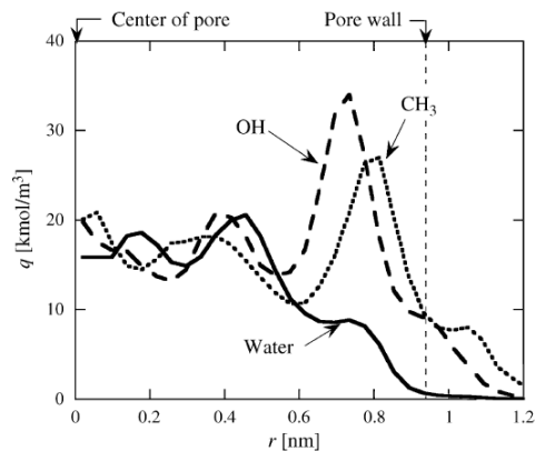
Fig. 4 Profils de densité de l'eau et du méthanol (groupements -OH et -CH_3 ) dans un pore d'une silice mésoporeuse fonctionnalisée par des fonctions triméthylsilyles ; T = 333 K et p/p_{0,pure} = 0,48 [17].
