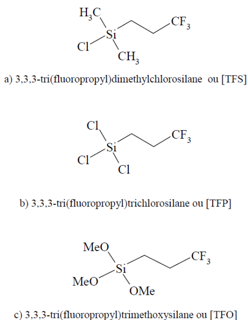
Fig. 2 Exemples de greffons fluorés couramment utilisés pour rendre une silice mésoporeuse hydrophobe [14].
