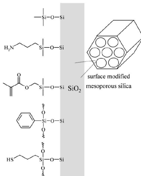
Fig. 3 Exemple de groupements fonctionnels pouvant être utilisés pour modifier les propriétés de surface d'une silice mésoporeuse [16].
