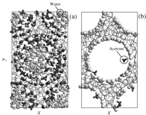
Fig. 5 Simulation de la répartition des molécules d'un mélange eau (molécules grises) et acétone (molécules noires) dans un pore portant des groupements de surface silanols (a) ou triméthylsilanes (b); T = 293 K, fugacité f = 12,6 kPa [17].
