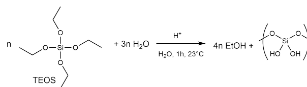
Fig. 8 Equation bilan de l'hydrolyse du TEOS.
