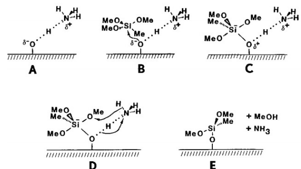
Fig. 6 Mécanisme proposé pour la réaction de silylation de surface d'une silice en présence d'une amine [7].
