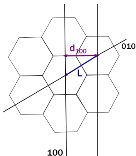
Fig. 13 Maille cristalline hexagonale 2D de la silice SBA-3 et paramètres pour la DRX.
