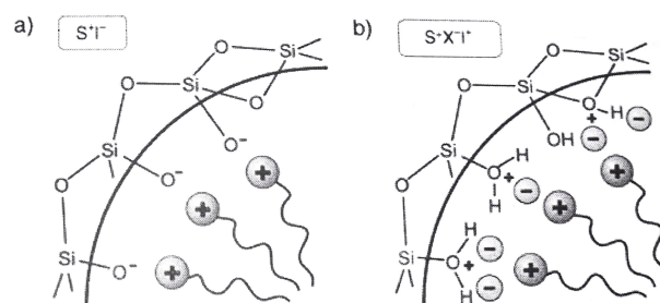
Fig. 9 Interfaces des silices mésoporeuses MCM-41 (a) et SBA-3 (b) [33].
