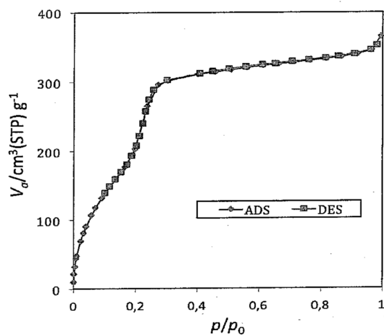
Fig. 15 Isothermes d'adsorption de N_2 à 77 K de la silice silylée ( S_{BET} = 1170 \text{ m}^2/\text{g} , C = 18 , V_{meso} = 0,50 \text{ cm}^3/\text{g} , dp = 2,2 \text{ nm} ).
