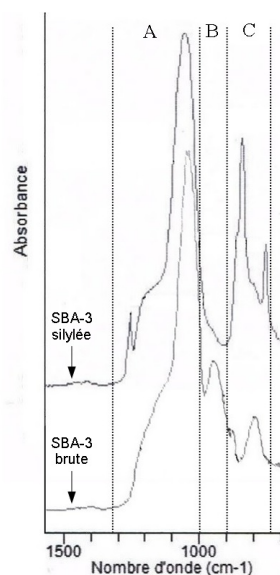
Fig. 11 Spectres IR d'un échantillon de SBA-3 avant et après la réaction de silylation.
