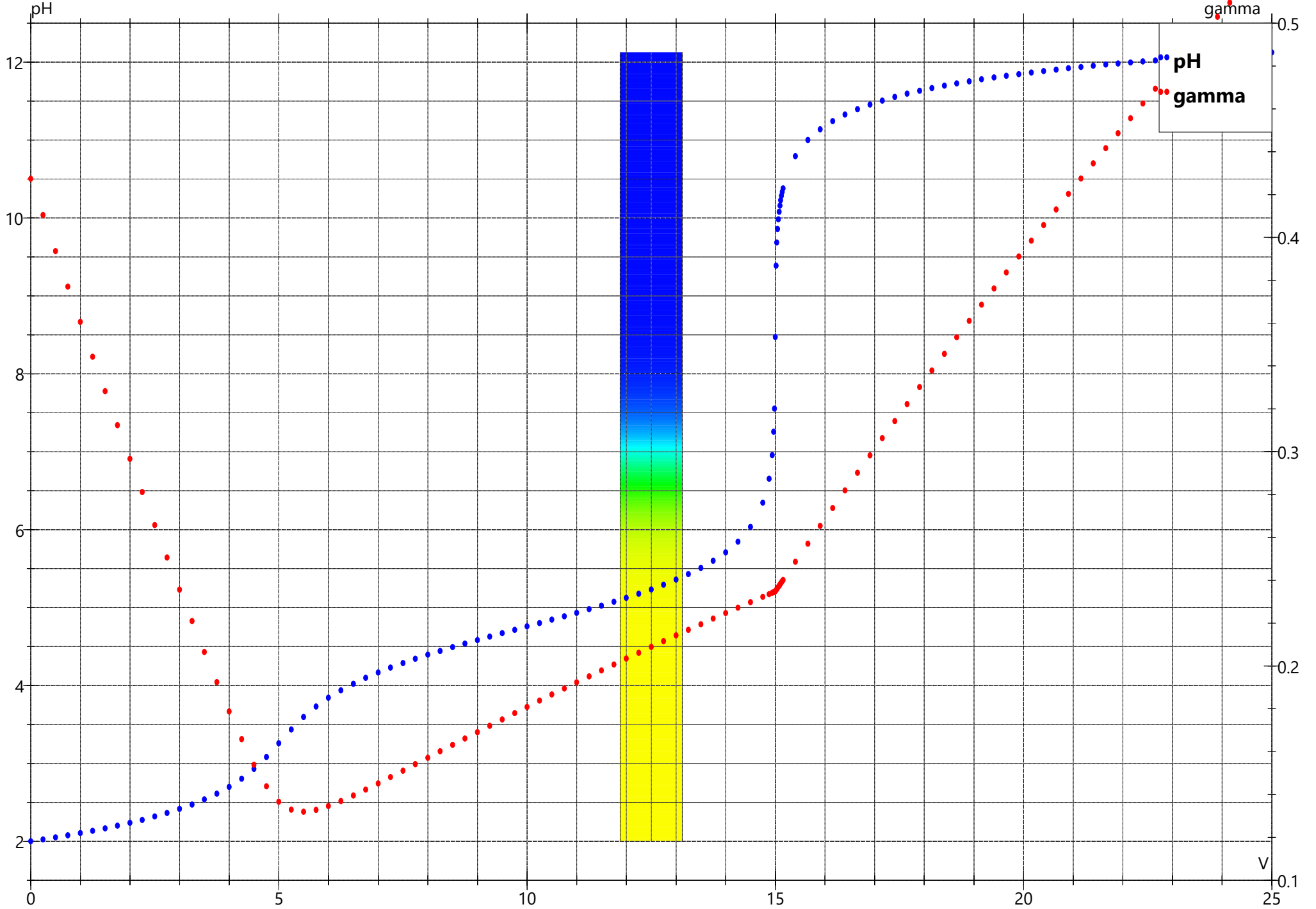
Dosage de 50mL de HCl(aq) (0.01 mol/L), Acide éthanoïque(aq) (0.02 mol/L), par 25mL de OH - (0.1 mol/L), Na + (0.1 mol/L)
