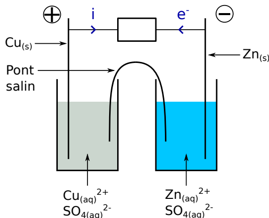
FIGURE 1 – Schéma de principe de la pile Daniel (source De la salle)
