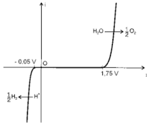
FIGURE 3 – Schema de principe des courbes IE (source Monnet)
