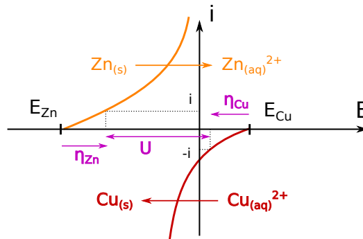
FIGURE 2 – Schema de principe des courbes IE (source De la salle)
