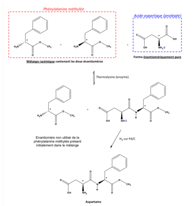
FIGURE 5 – Synthèse industrielle de l'aspartame - source Eduscol
