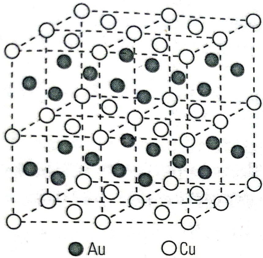
Fig. 1 – CuAu.
