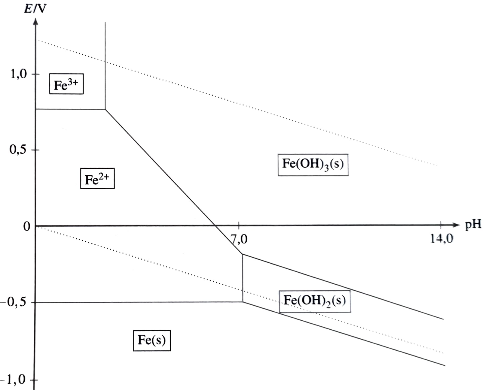
FIGURE 10.4 – Diagramme E -pH du fer
