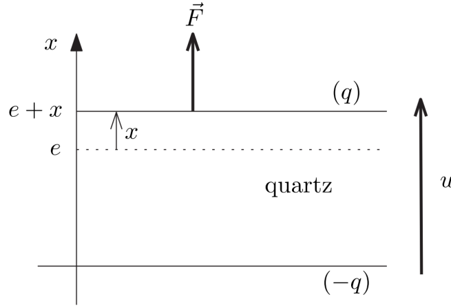
FIGURE 5 – Schéma du condensateur en quartz
