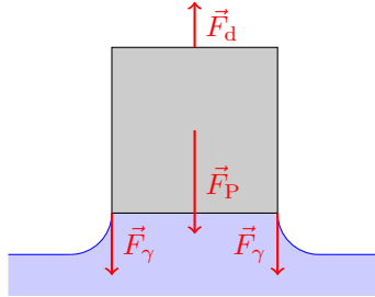
FIGURE 14 – Une plaque en surface d'un liquide est soumise à son propre poids et aux forces capillaires, verticales à la limite d'arrachement.
