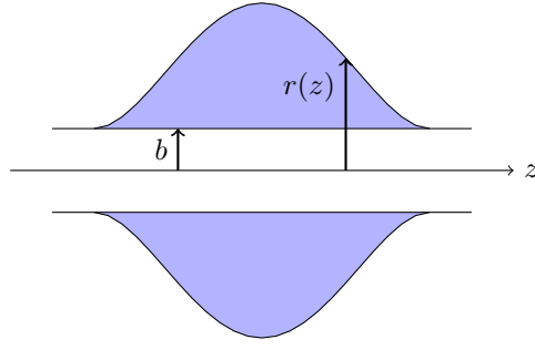
FIGURE 3 – Une goutte d'un liquide est posé sur un cylindre de rayon b . En l'absence de pesanteur, la goutte adopte une forme dite ondoïdale.
