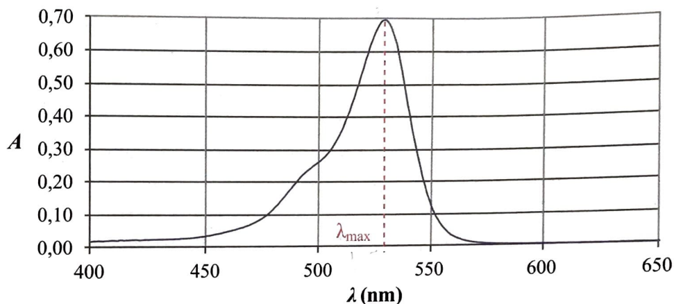
Figure 1 – Spectre UV-visible de l'érythrosine B dans l'eau
