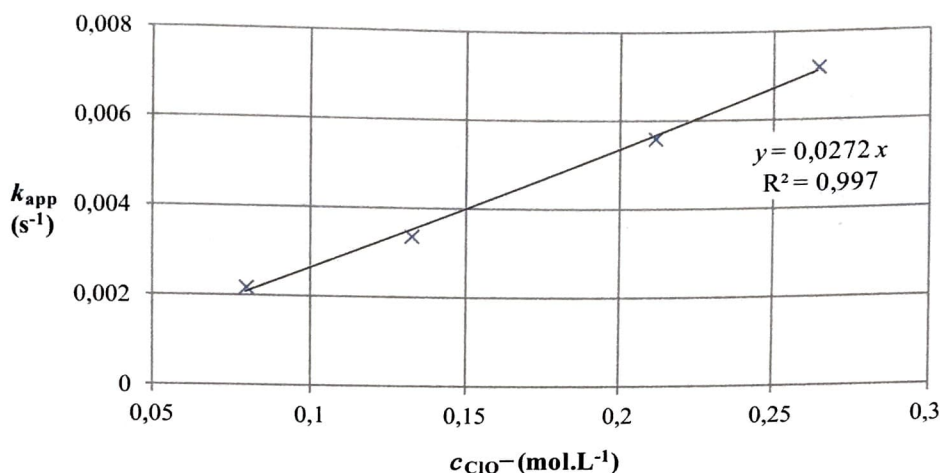
Figure 5 – Évolution de la constante cinétique apparente avec la concentration en ClO^-
