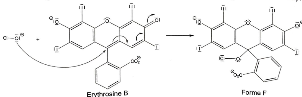
Figure 2 – Réaction des ions hypochlorite sur l'érythrosine B
