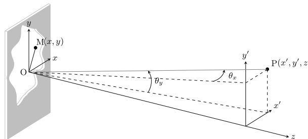
FIGURE 3 – Adapté de physagreg.com . Paramétrisation de l'intensité en un point après passage de la lumière dans un objet diffractant.
