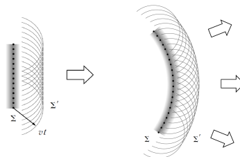
FIGURE 1 – Source : Clément de la Salle. En propagation libre, le principe de Huygens Fresnel est valide : une onde plane reste plane, une onde sphérique reste sphérique
