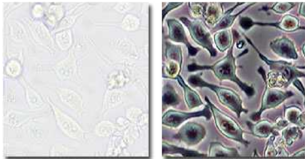
FIGURE 4 – Image de cellules : microscope classique (à gauche) et microscope à contraste de phase (à droite)
