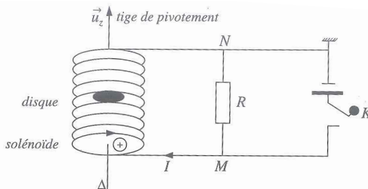
FIGURE 7 – Générateur alimentant un solénoïde entouré d'un isolant chargé.
