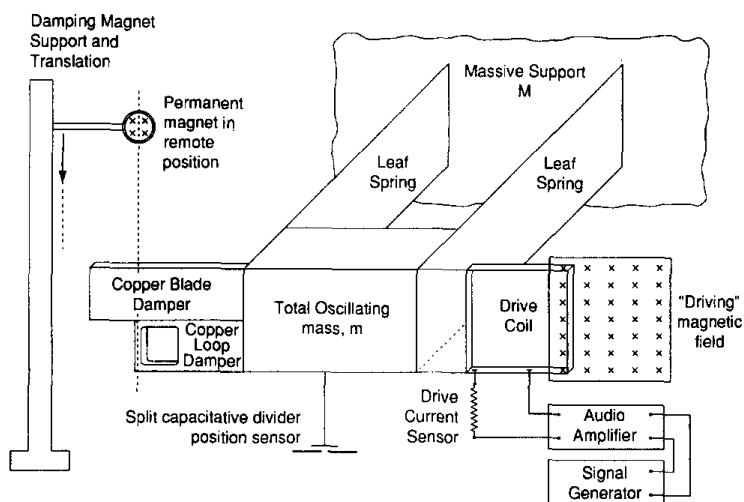
FIGURE 5 – Une masse ( total oscillating mass ) couplée à des ressorts ( leaf spring ) oscille sous l'action d'un forçage monochromatique exercé par un système magnétique ( driving magnetic field ) dont on ne décrira pas le principe de fonctionnement. L'amortissement est contrôlé par un système de friction magnétique ( dampers+damping magnets ).
