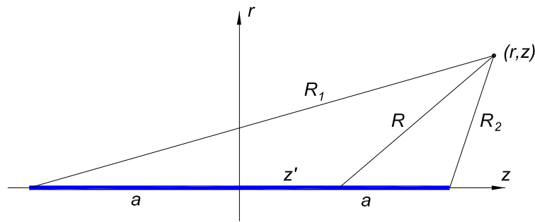
FIGURE 8 – Aiguille chargée de taille 2a . La goutte d'eau chargée est située en (r, z) (base cylindrique).
