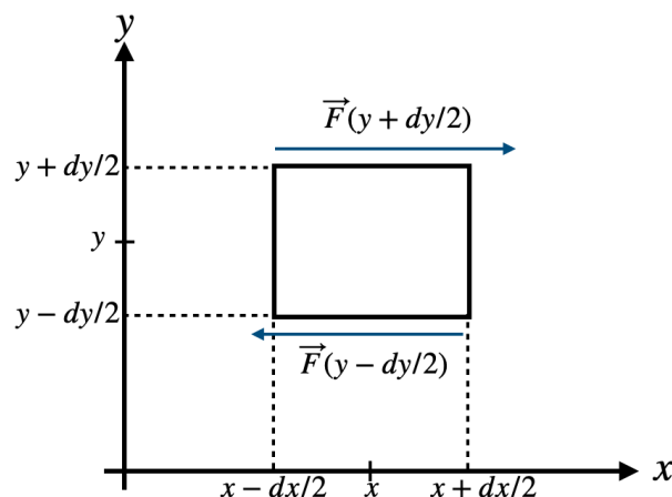
FIGURE 2 – Particule de fluide soumise à des contraintes de cisaillement
