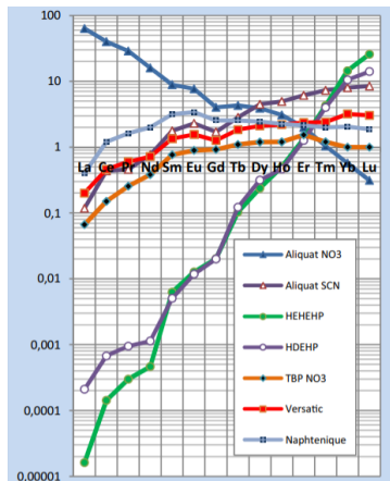
Figure 1: Facteur de séparation pour différents agents d'extraction
