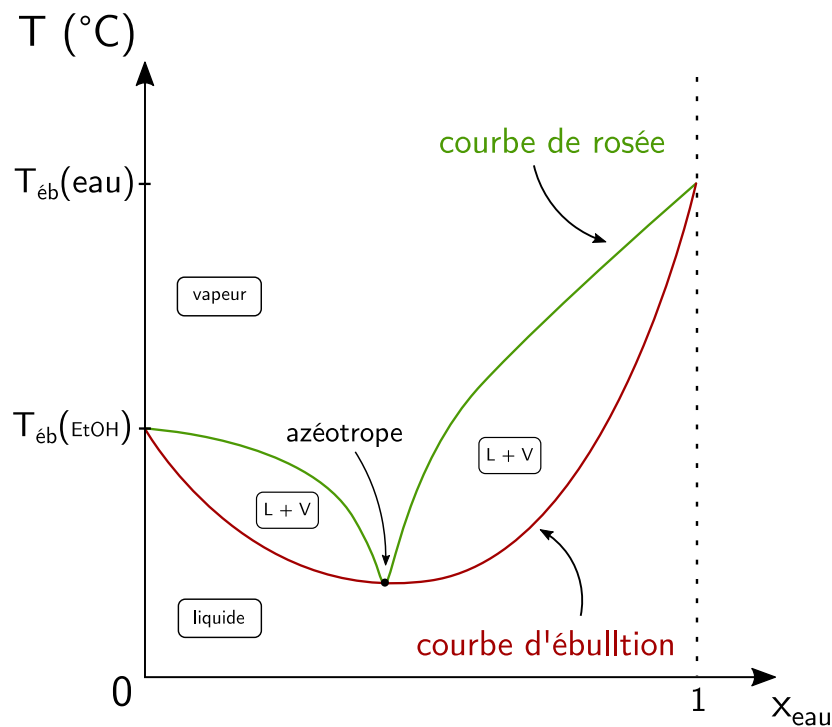
Fig. 2 : Mélange binaire avec azéotrope
