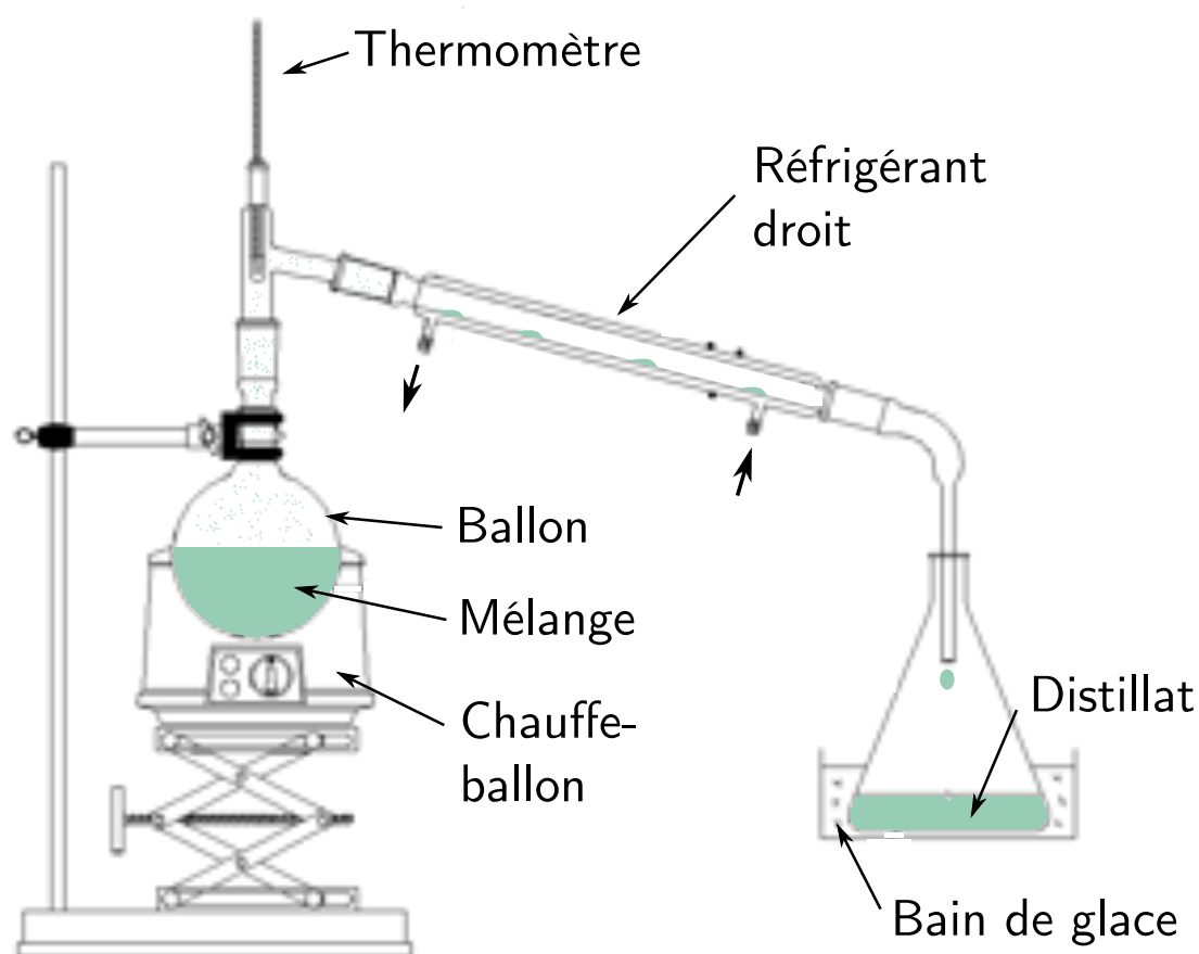
Fig. 3 : Schéma de montage de distillation
