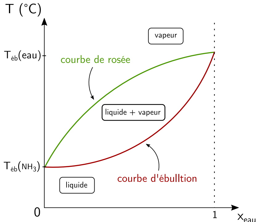
Fig. 1 : Diagramme binaire d'un mélange idéal
