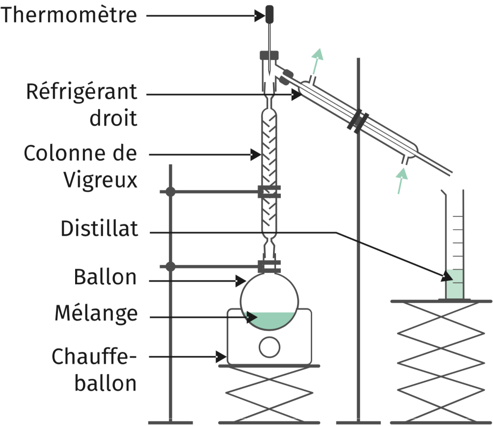
Fig. 4 : Schéma de montage de distillation fractionnée
