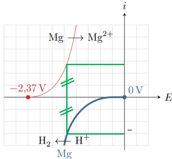
Fig. 5 : Point de fonctionnement pour la corrosion du magnésium
