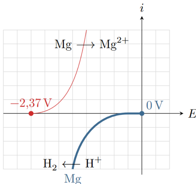
Fig. 4 : Courbes intensité potentiel correspondant à la corrosion du magnésium
