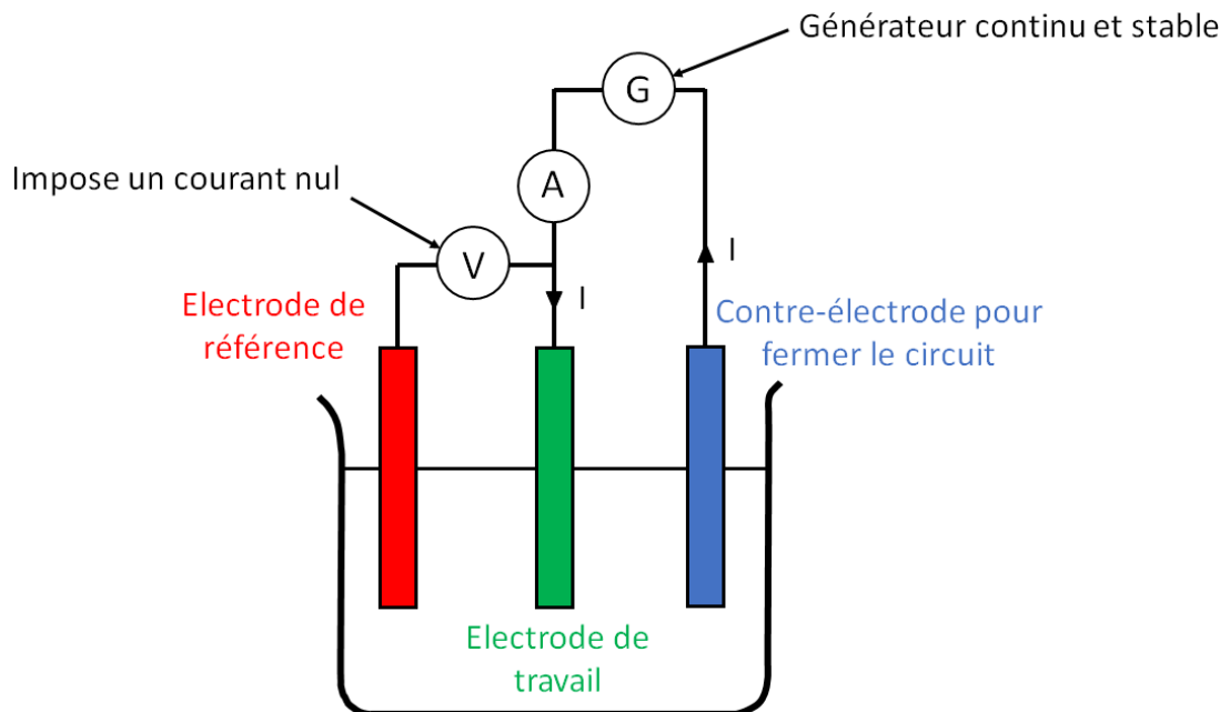
Fig. 3 : Montage à trois électrodes
