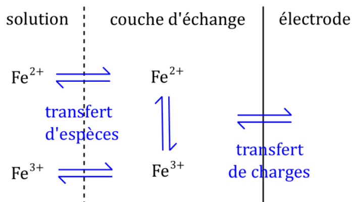
Fig. 1 : Lieu des échanges lors d'une réaction électrochimique à une électrode
