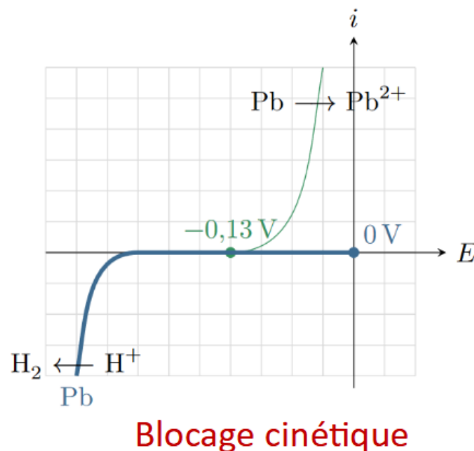
Fig. 6 : Blocage cinétique pour la corrosion du plomb
