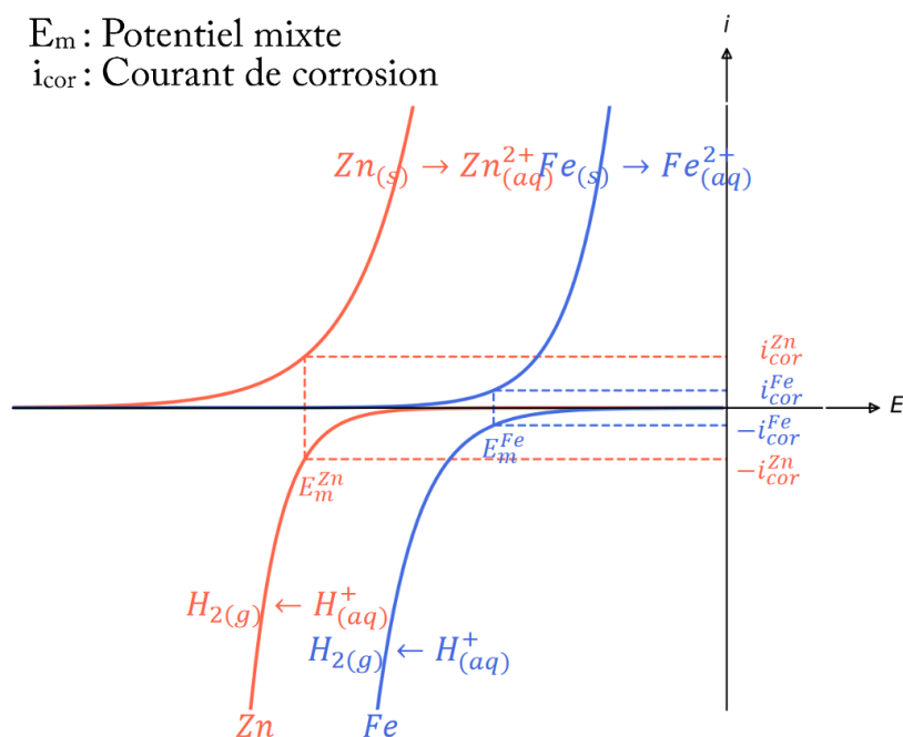
Fig. 7 : Courbes d'oxydation et de réduction pour le fer et le zinc.
