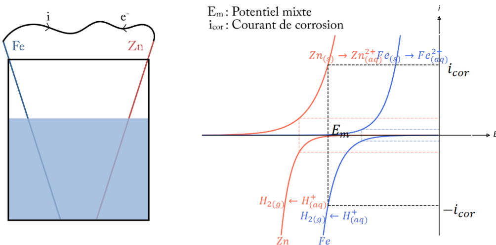
Fig. 8 : Point de fonctionnement du système lorsque fer et zinc sont en contact.
