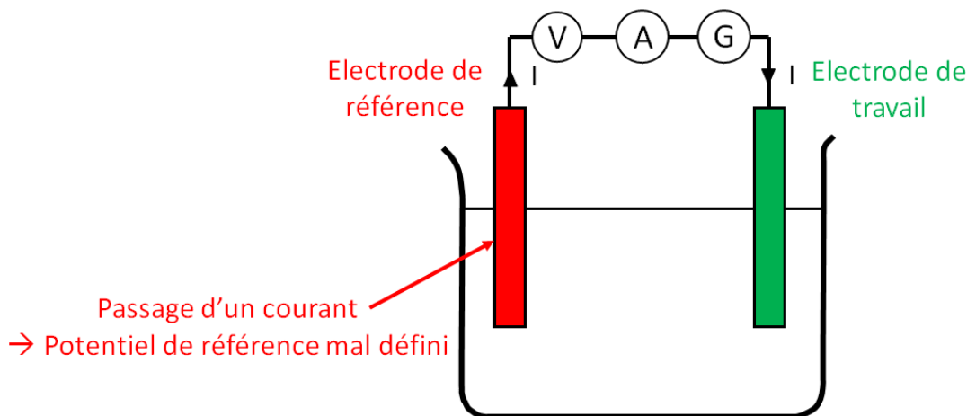
Fig. 2 : Montage à deux électrodes
