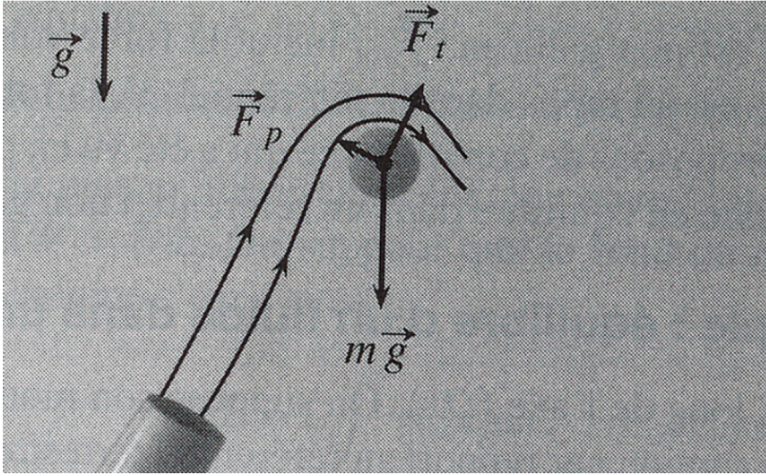
FIG. 1 : Les lignes de courants passent sur la balle, la pression y augmente et la balle se retrouve maintenue dans les airs.
