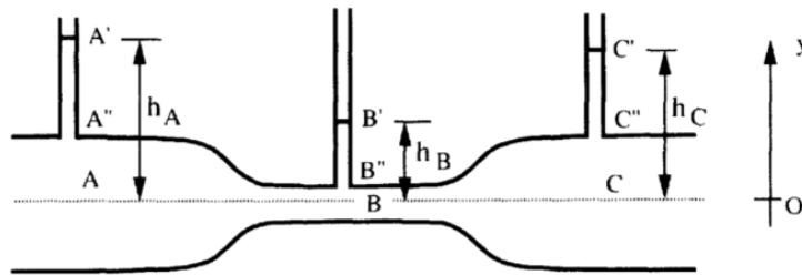
FIG. 3 : Effet venturi
