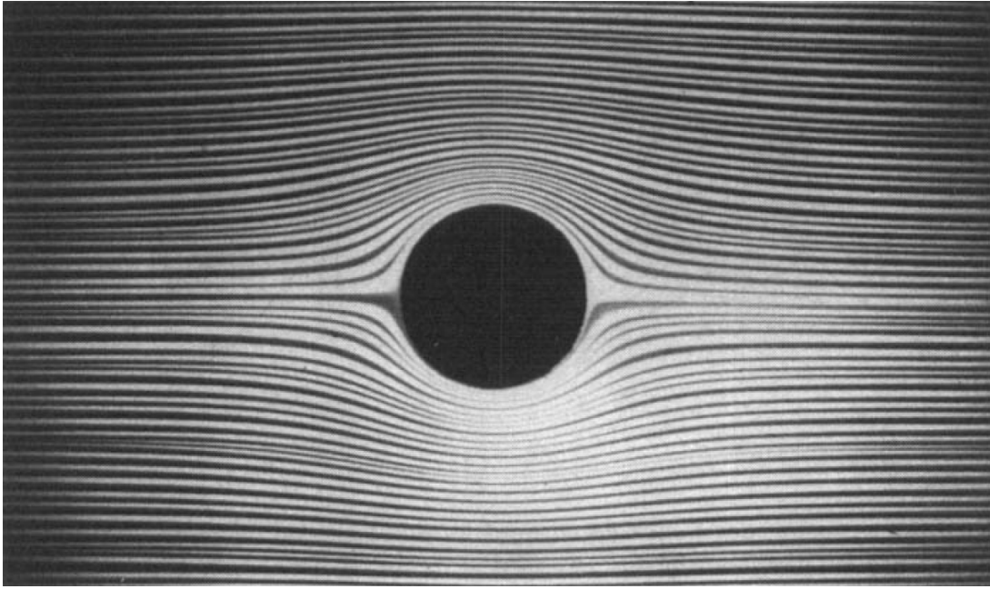
FIG. 4 : Forme des lignes de courant dans le cas d'écoulement parfait autour d'un cylindre sans rotation.
