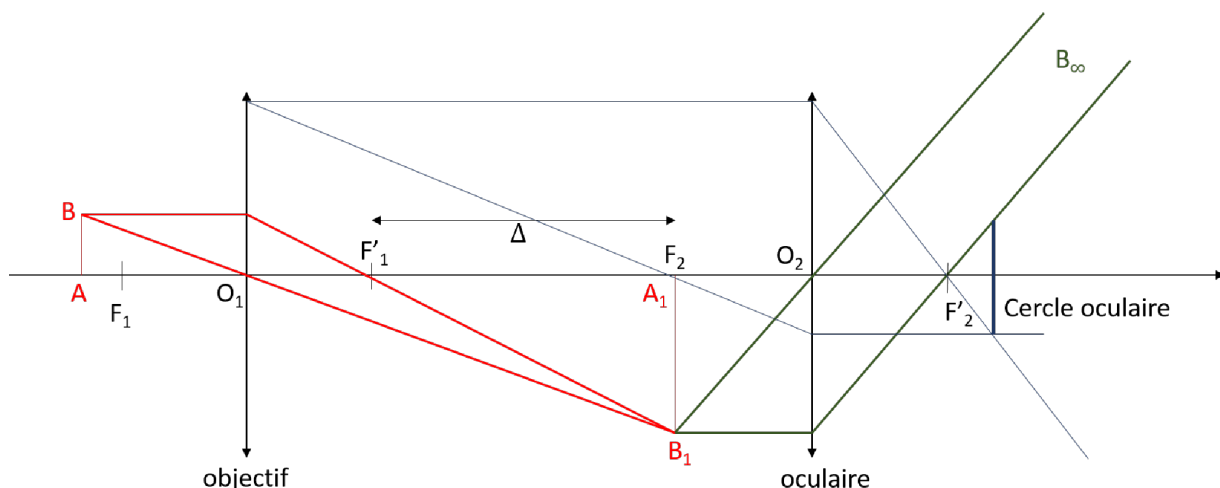
FIG. 1 : Schéma du microscope à deux lentilles
