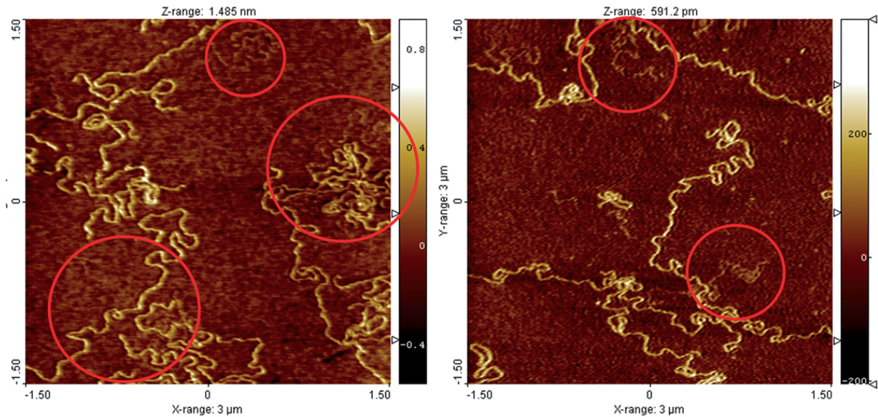
FIG. 5 : Image d'ADN double brin et simple brin faite avec un microscope en champ proche à l'EPFL
