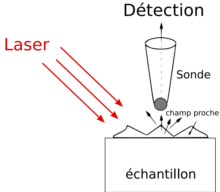
FIG. 4 : Principe de fonctionnement d'un microscope à champ proche
