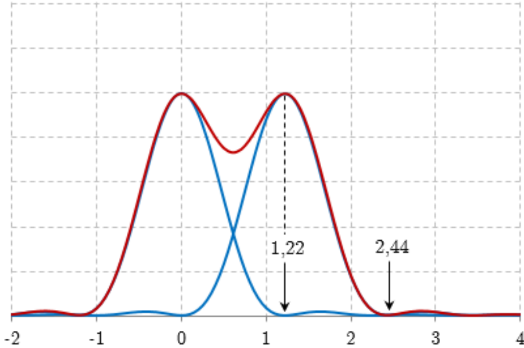
FIG. 2 : Profil d'intensité pour deux taches tout justes distinguables selon le critère de Rayleigh
