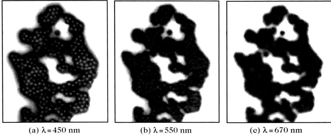
FIG. 3 : Billes de latex de 500 nm de diamètre recouvertes d'or observées au microscope optique à différentes longueur d'ondes.
