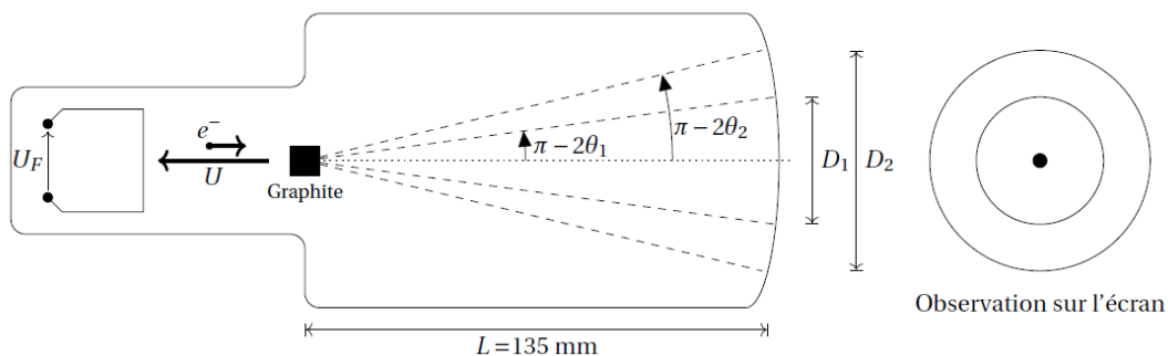
FIG. 7 : Dispositif expérimental
