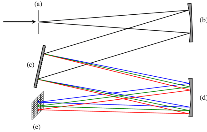
FIG. 3 : Schéma d'un spectro à réseau à réflexion
