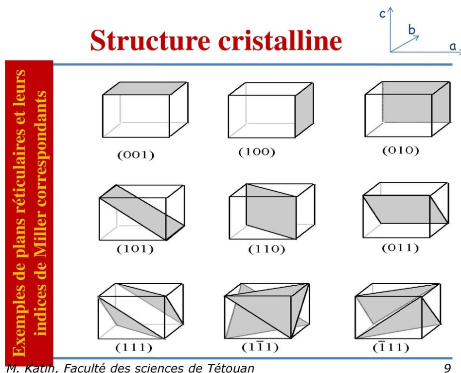
FIG. 4 : Exemples de plans réticulaires et indices de Miller associés.
