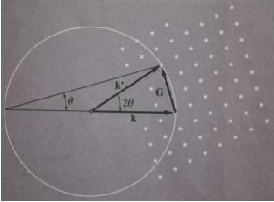
FIG. 6 : Sphère d'Ewald. Les points blancs sont des noeuds dans le RR du cristal. On place l'extrémité du vecteur d'onde incident \vec{k}_0 sur l'un des noeuds. On trace une sphère de rayon 2\pi/\lambda autour de l'origine de \vec{k}_0 . Si le cercle intercepte un autre noeud du RR alors on peut définir un \vec{k} respectant la condition de Von Laue.
