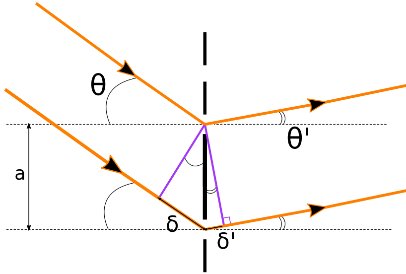
FIG. 2 : Configuration étudiée. Le faisceau incident arrive avec un angle \theta sur le réseau vertical.
