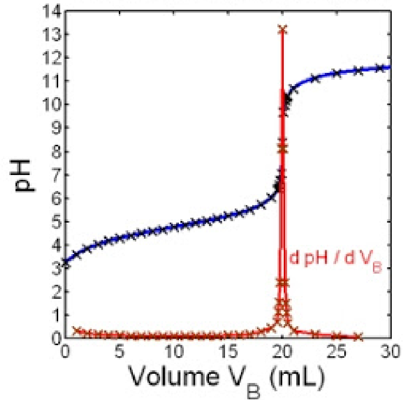
Méthode de la dérivée
