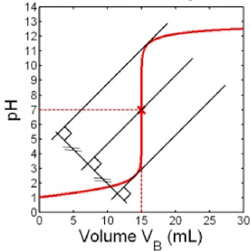
Méthode des tangentes
