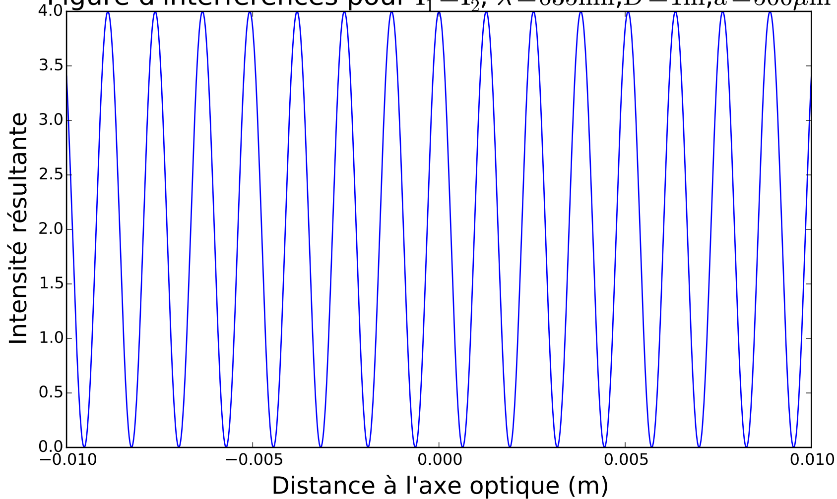
Figure d'interférences pour I_1 = I_2 , \lambda = 635\text{nm} , D = 1\text{m} , a = 500\mu\text{m}
