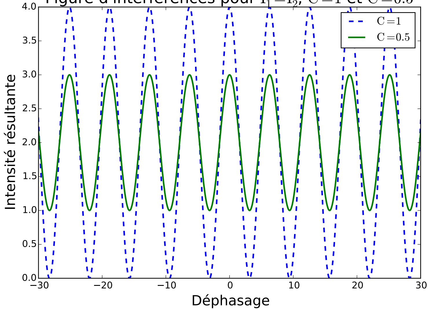
Figure d'interférences pour I_1 = I_2 , C = 1 et C = 0.5
