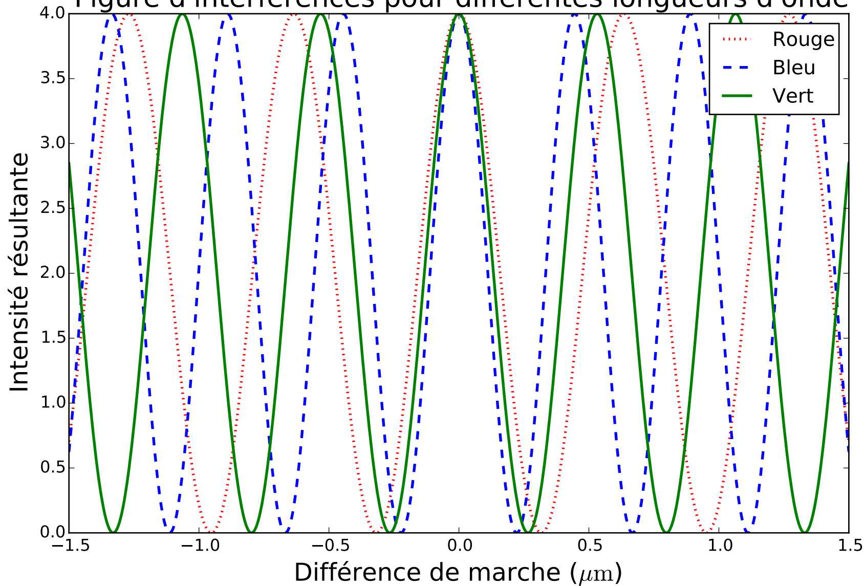
Figure d'interférences pour différentes longueurs d'onde
